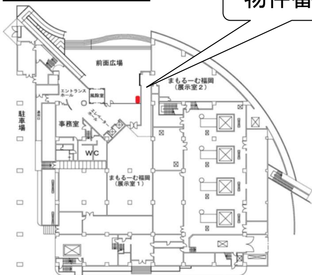
1 階 平 面 図
