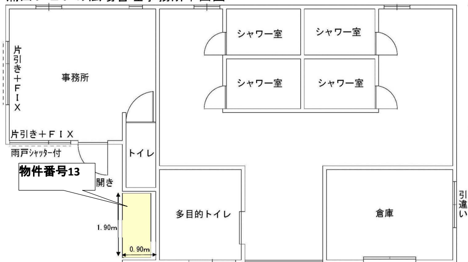
蒲田いこいの広場管理事務所平面図
