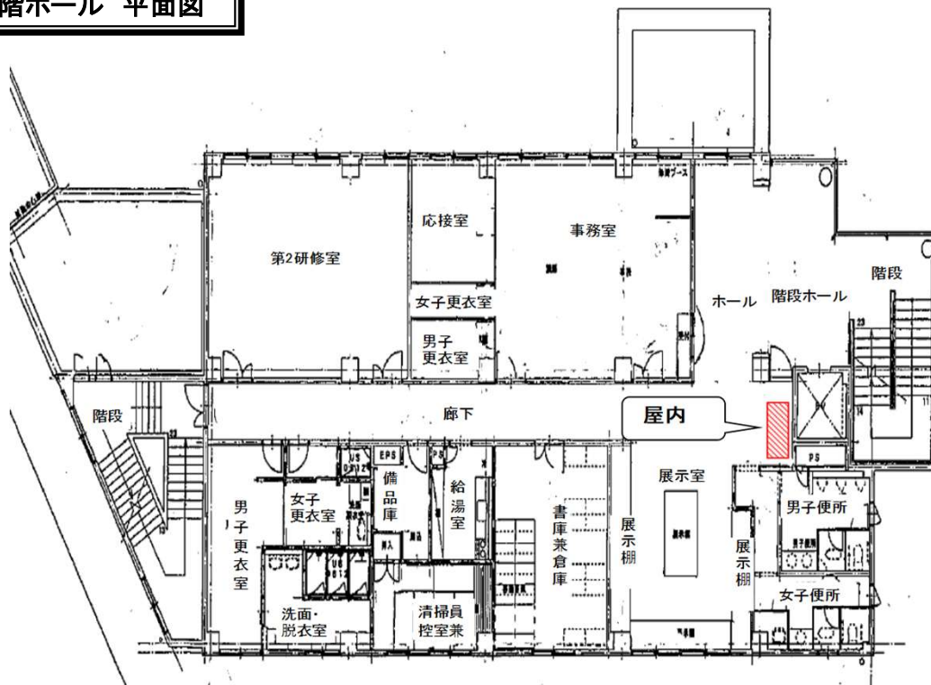
2階ホール 平面図
