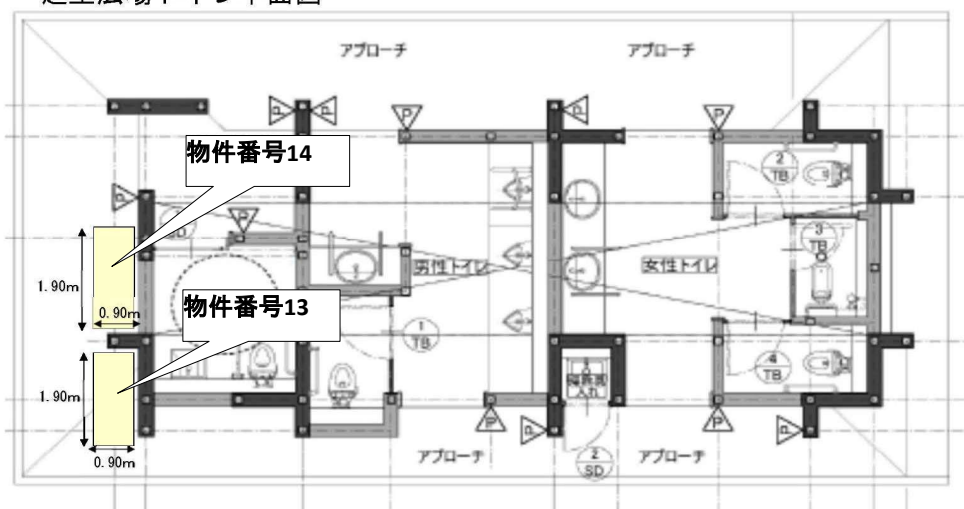
芝生広場トイレ平面図
