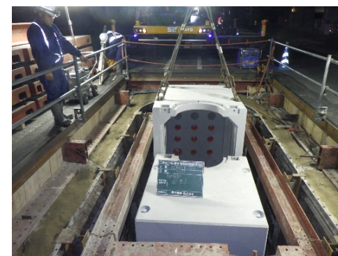
①特殊部施工状況
