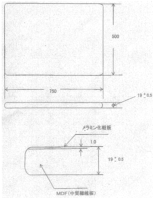
天板規格図
