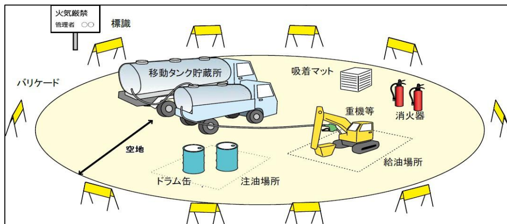
災害現場等における危険物の仮貯蔵・仮取扱いイメージ図（出典：総務省消防庁資料）
