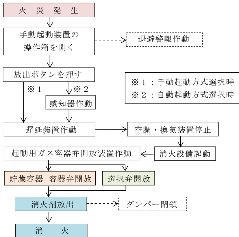
図 2 手動起動動作フロー
