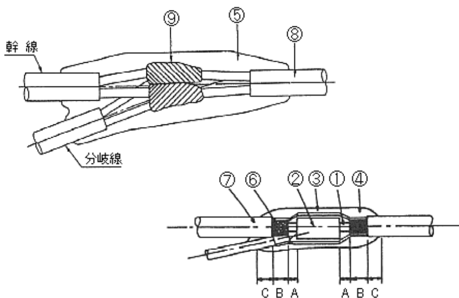
線心接続部拡大図
