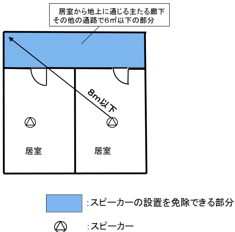
第 15－8 図 居室から地上に通じる主たる廊下その他の通路で免除できる場合
