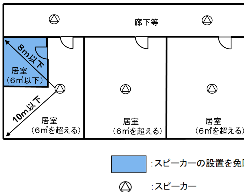
第15-7図 居室でスピーカーの設置を免除できる場合
