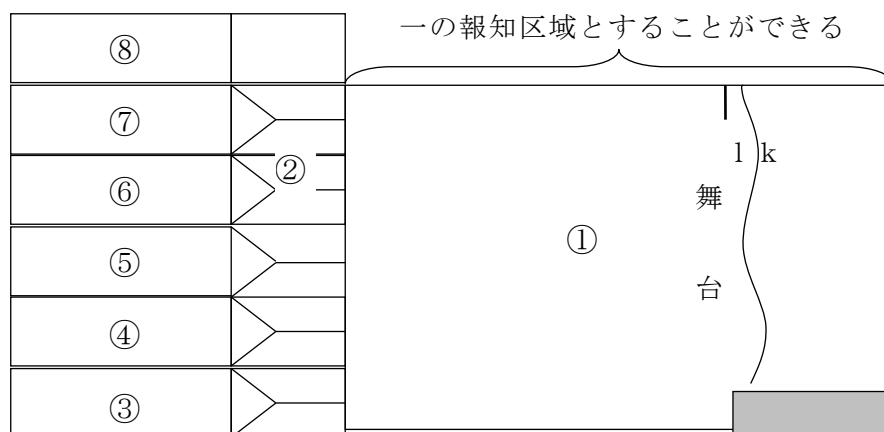
第 15－5 図（吹き抜けがある場合の報知区域の設定例）
