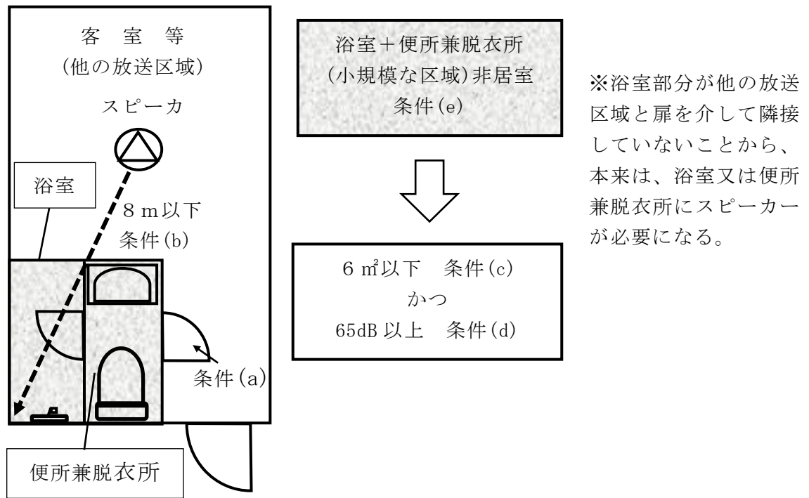
第 15-13 図 小規模な区域がある場合
