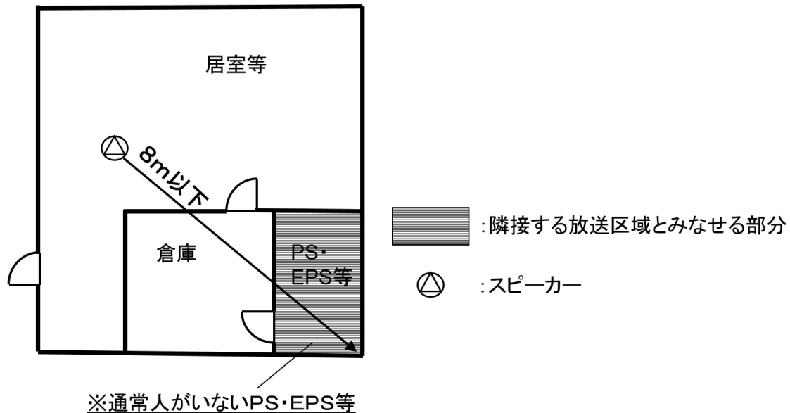
第15-12図 隣接していない放送区域がある場合
