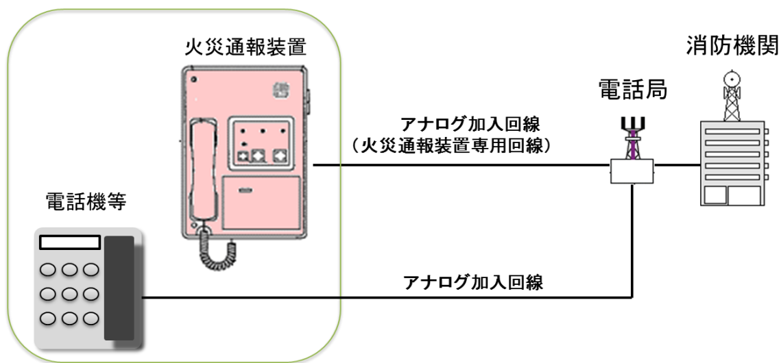
第 14-1 図 電話回線に専用回線で接続する火災通報装置の概要図
