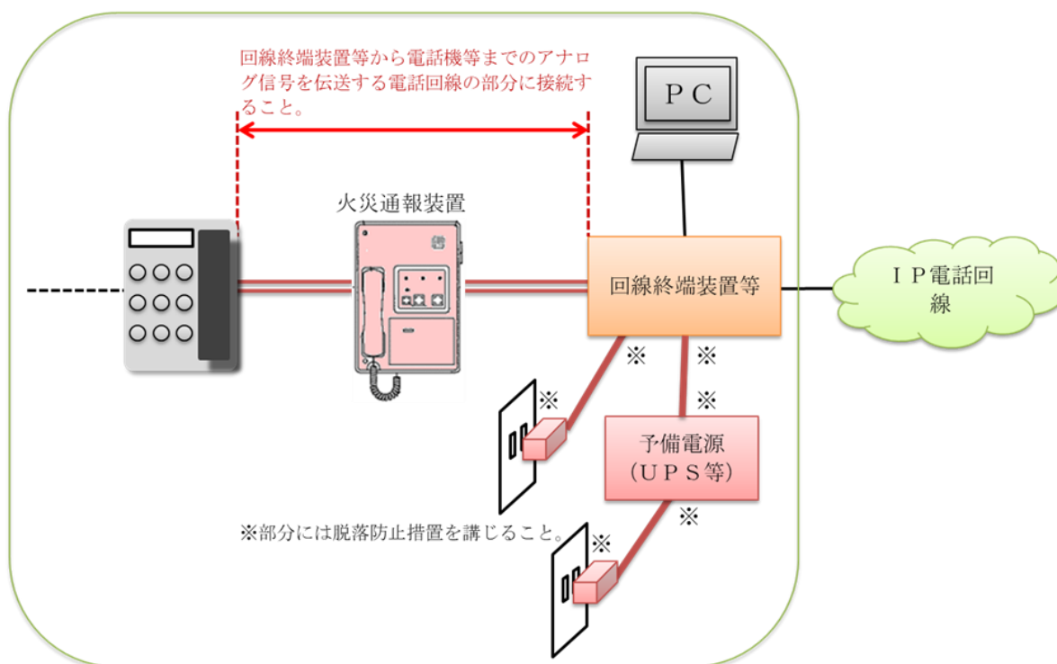
第14-6図 IP電話回線における火災通報装置の接続部分について
