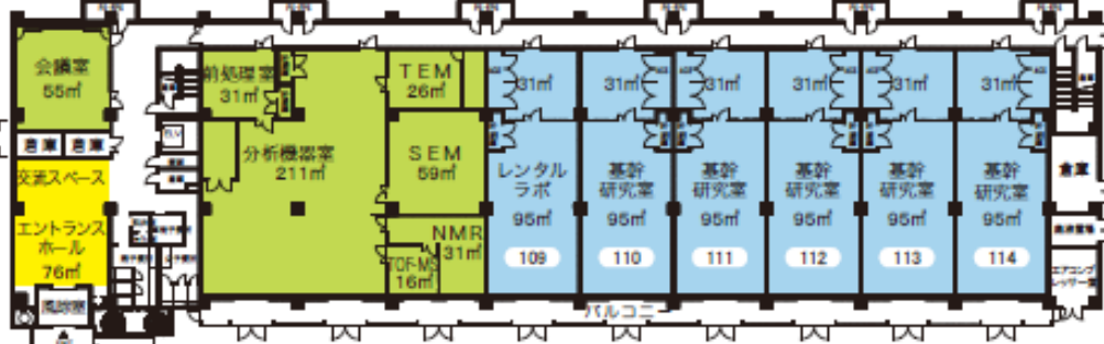
■ 1階平面図
