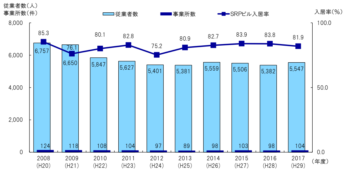
SRP 地区 36 関連企業集積(事業所数・従業員数, SRPビル入居率)
