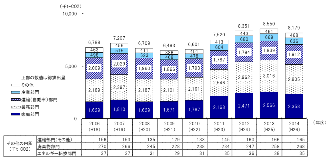
二酸化炭素排出量(部門別)(2014 年度)
