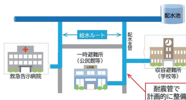
耐震ネットワーク工事の概要
