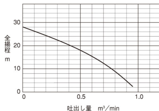
性能曲線
