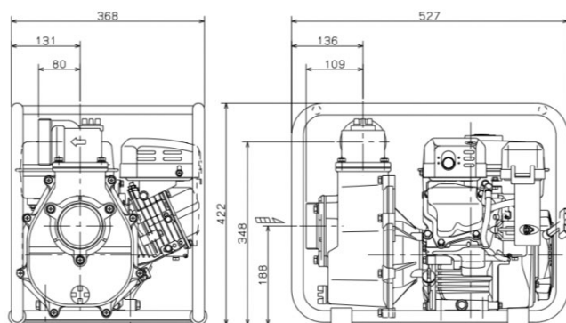
寸法図
