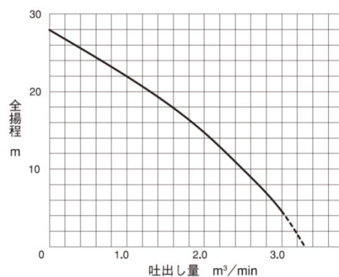
性能曲線
