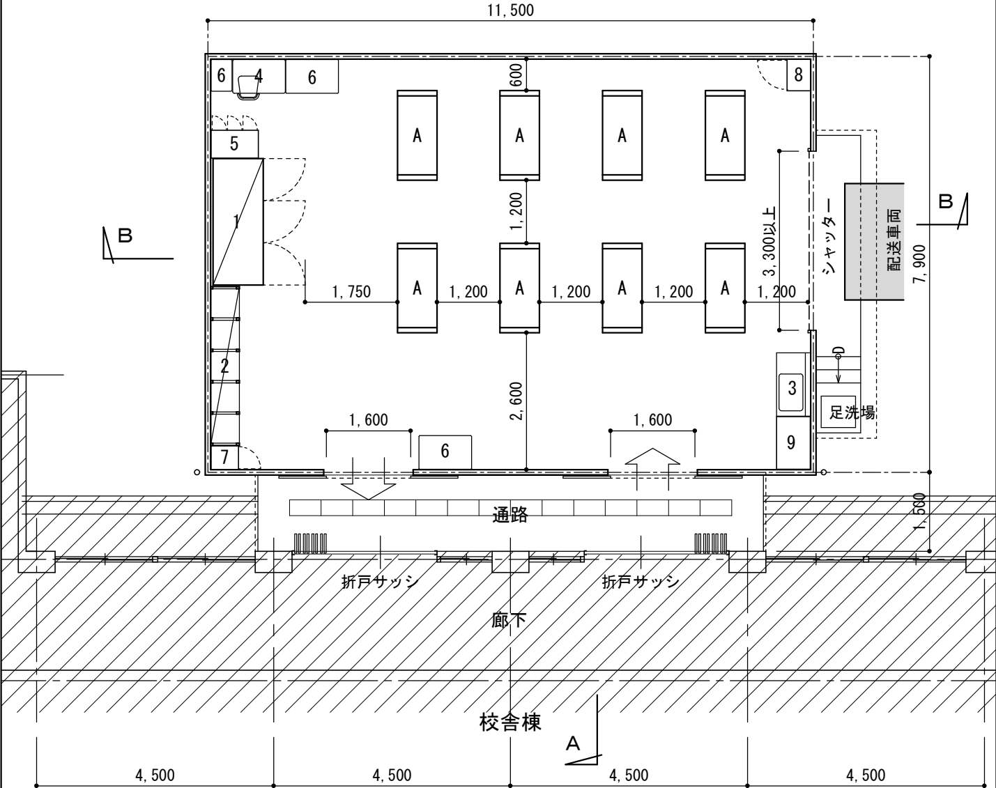
平面図 S=1:100
