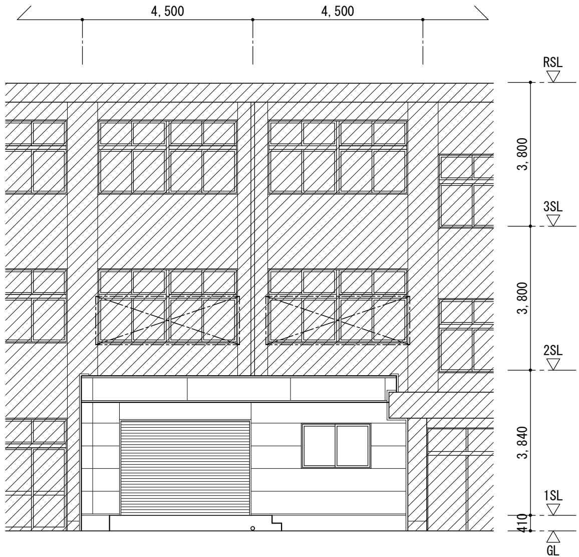
改修立面図
