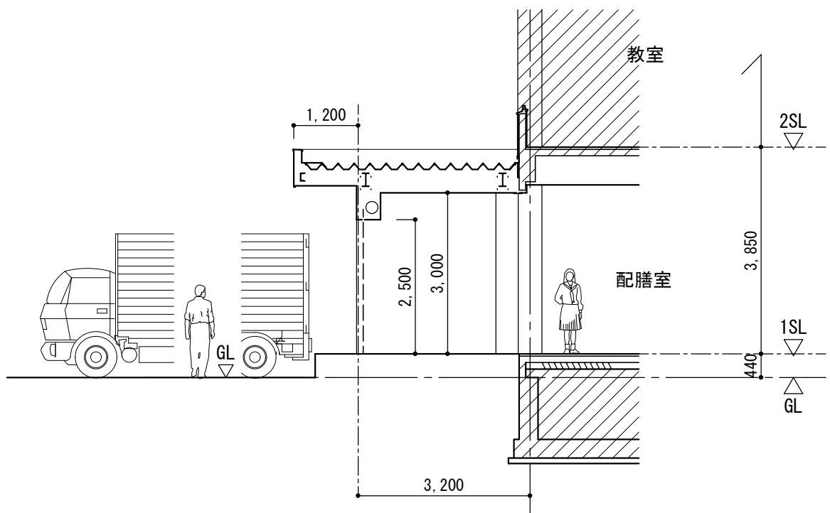
A-A 改修断面図
