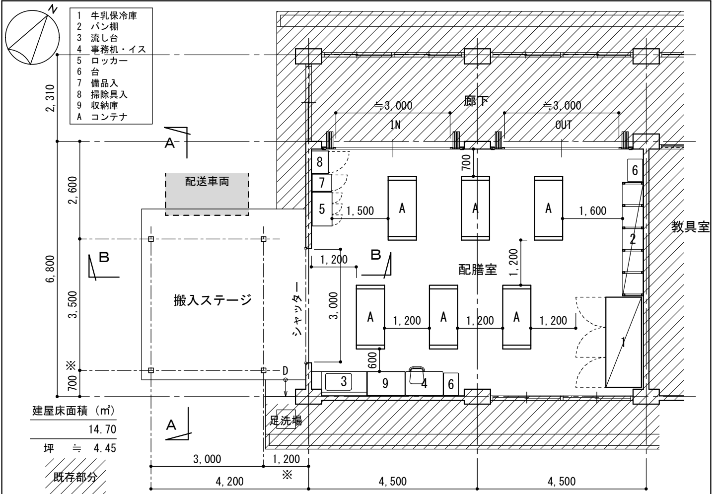
改修平面図
