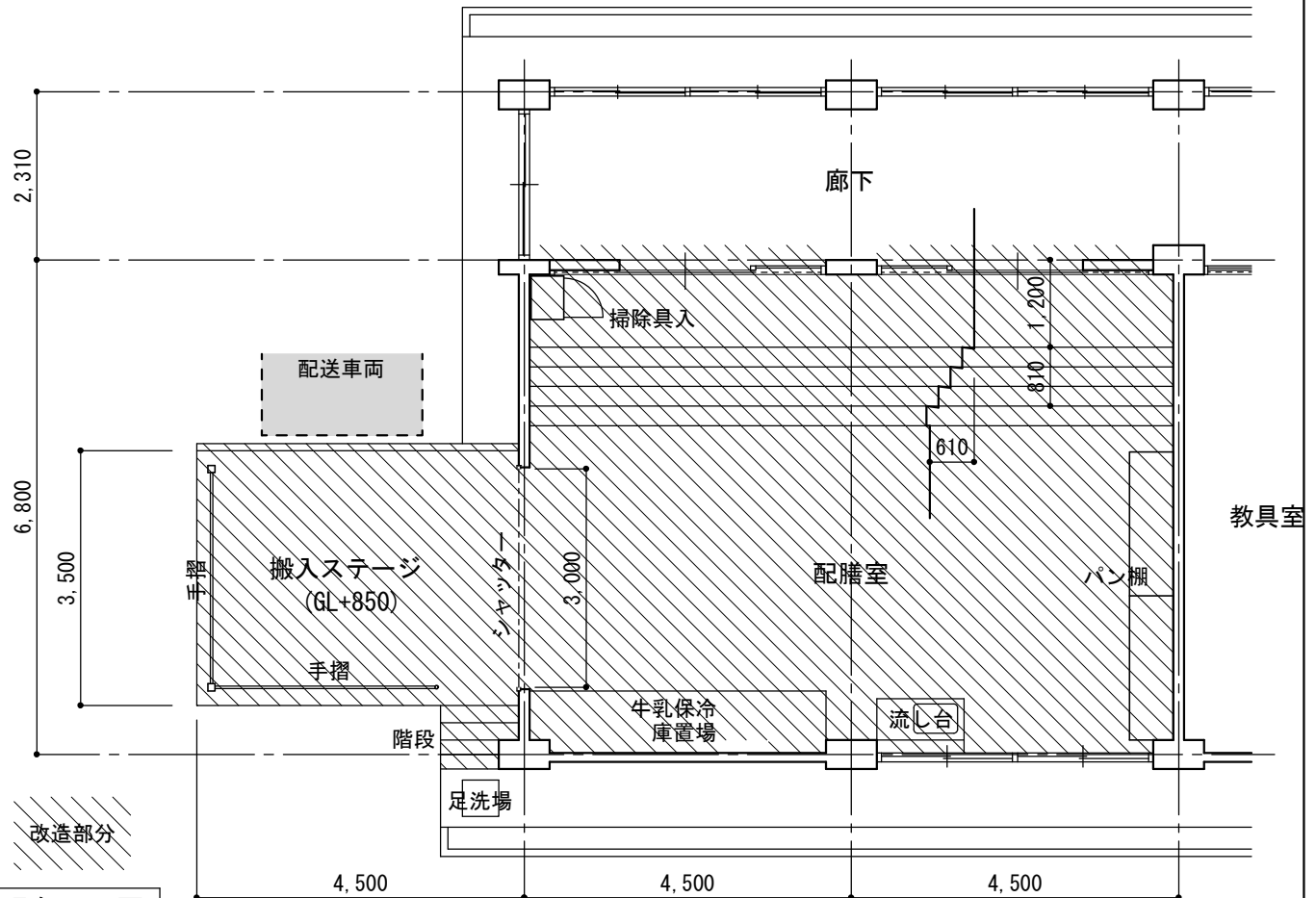
既存平面図
