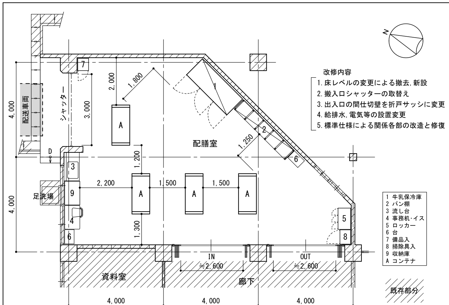
改修平面図
