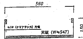
B 部断面図
