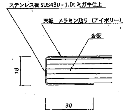
天板断面图
