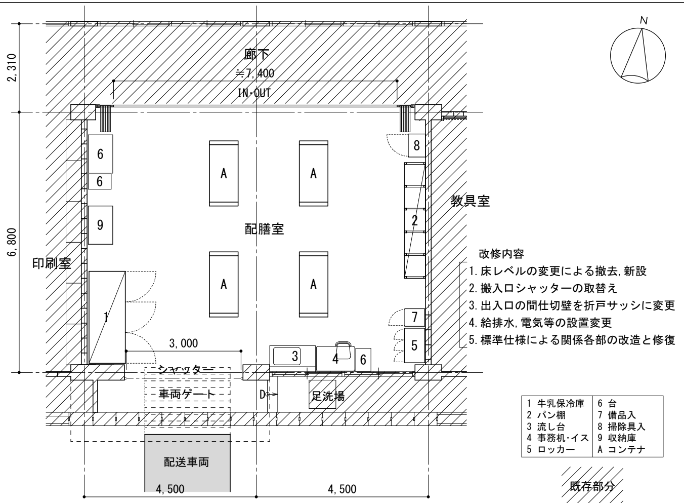
改修平面図
