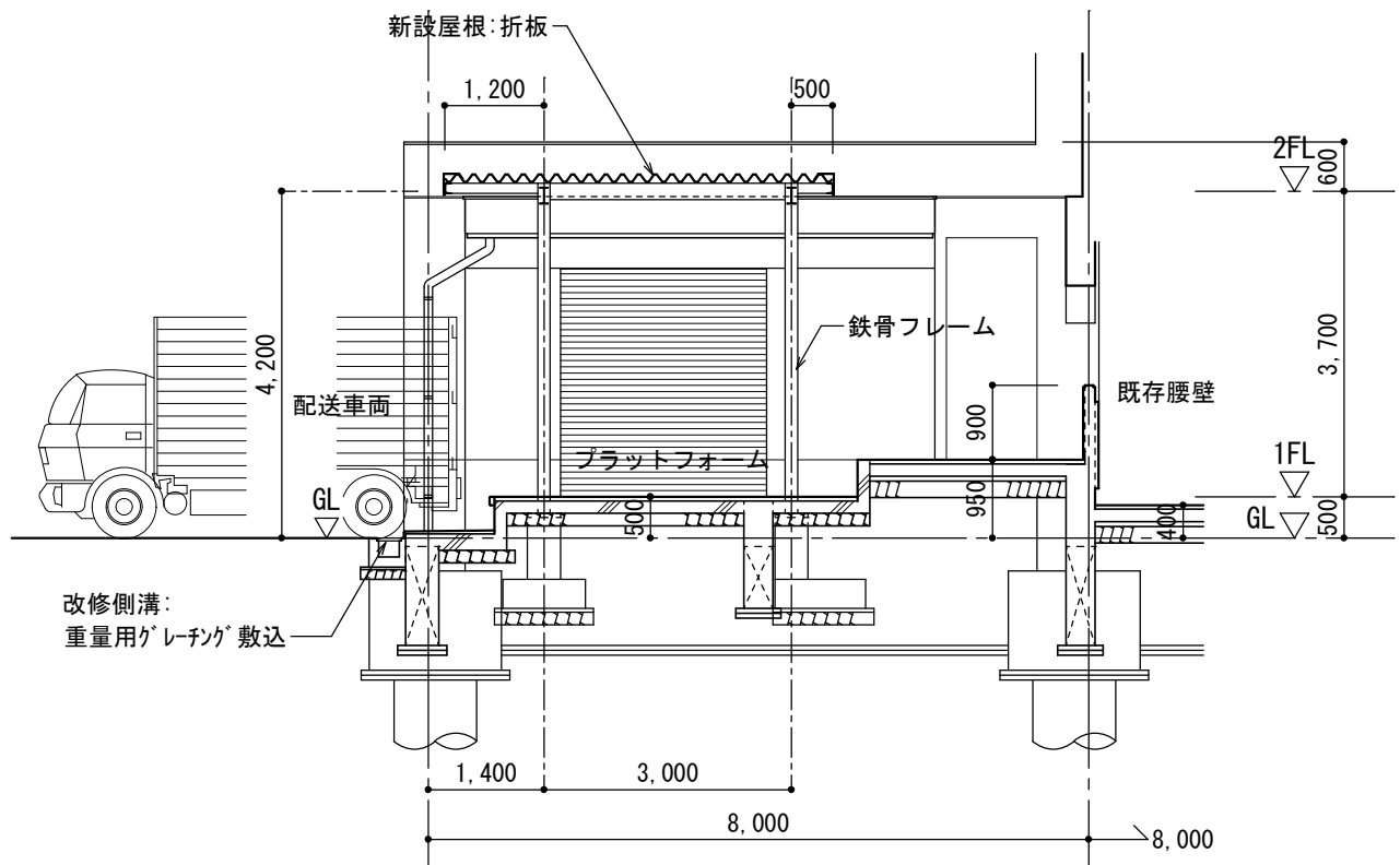
B-B断面図
