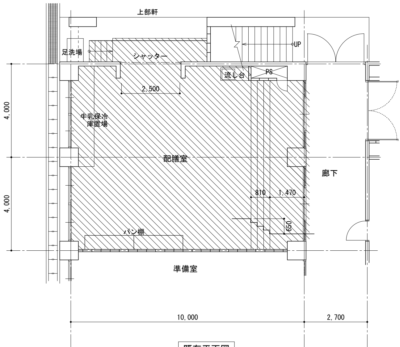
既存平面図
