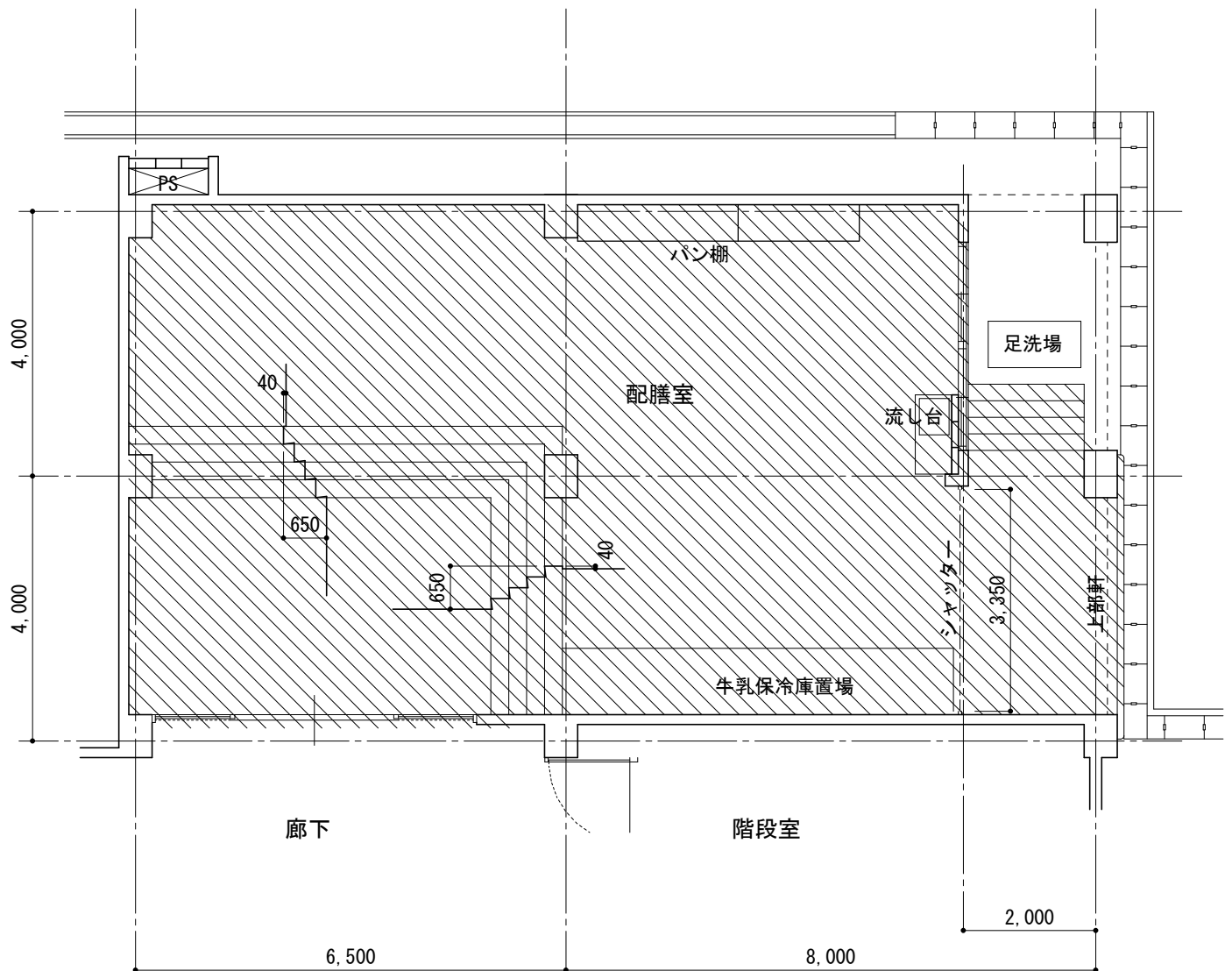
既存平面図
