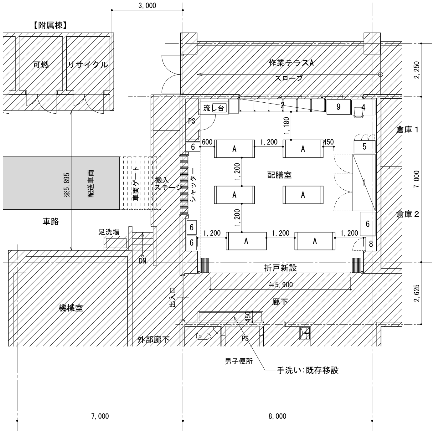
改修平面図
