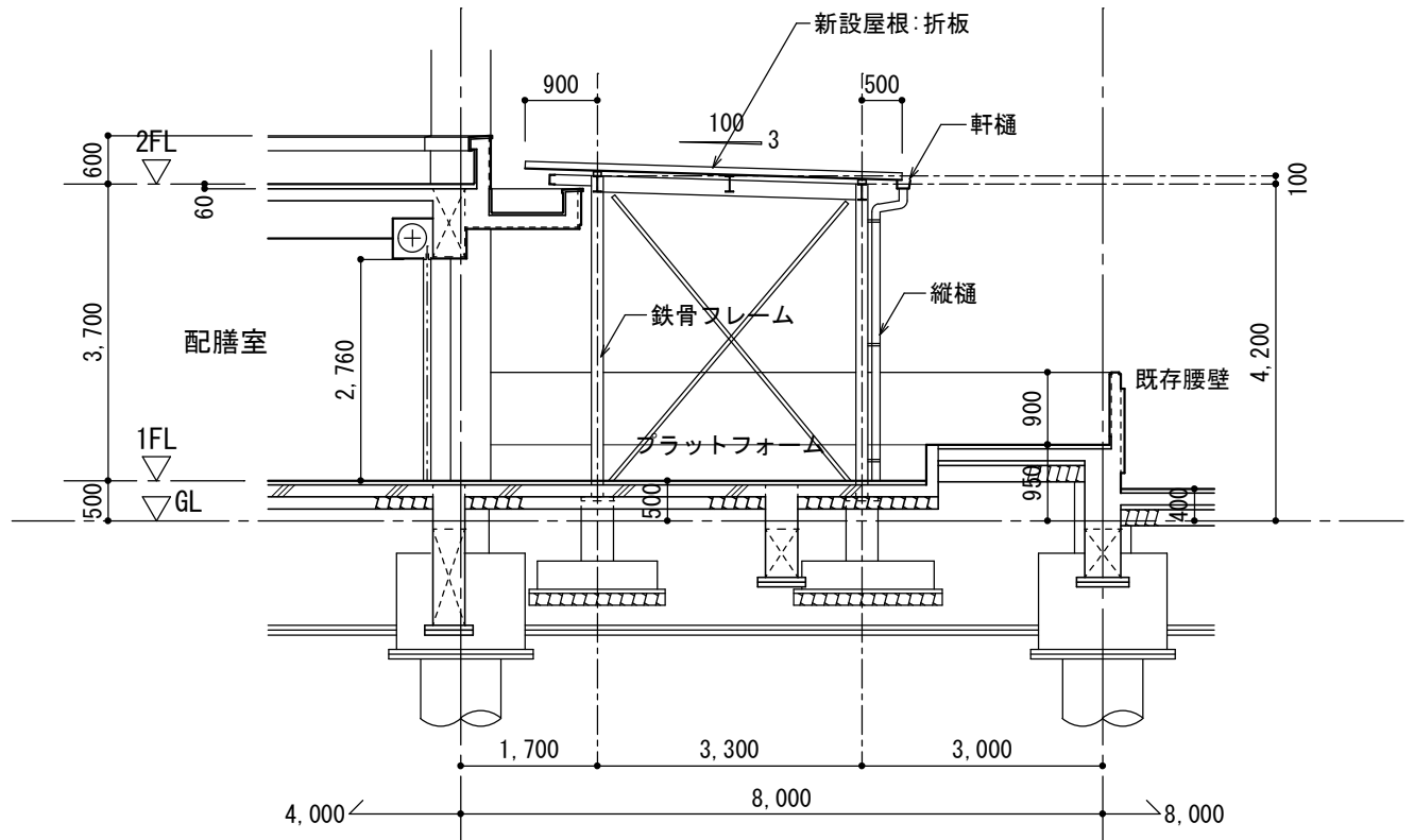
A-A断面図
