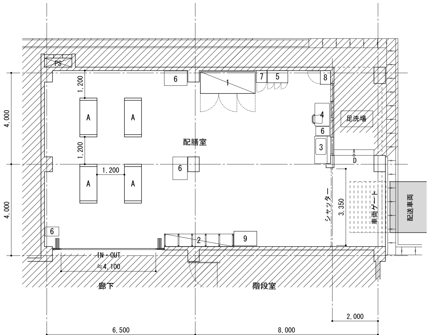
改修平面図
