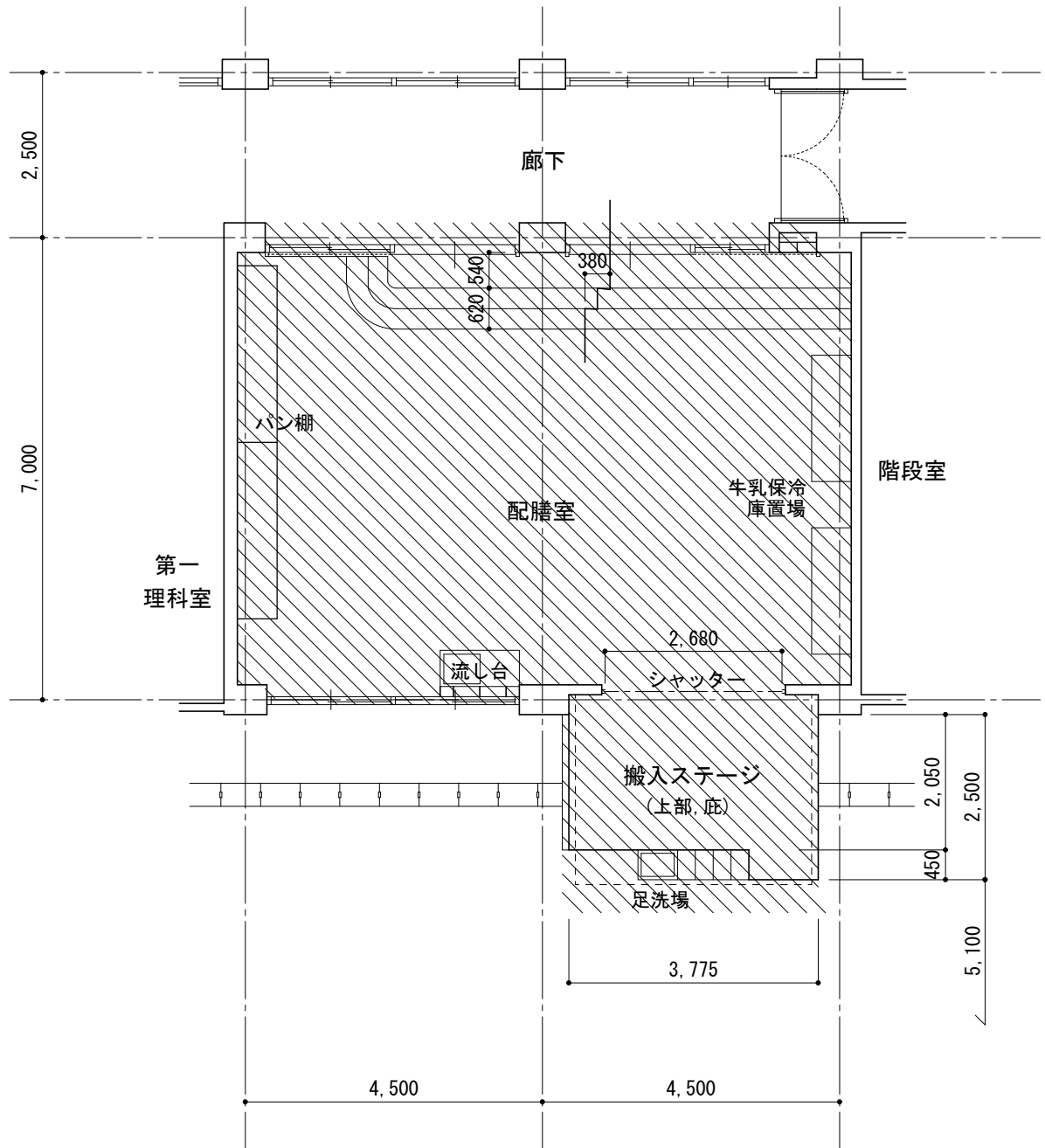
既存平面図
