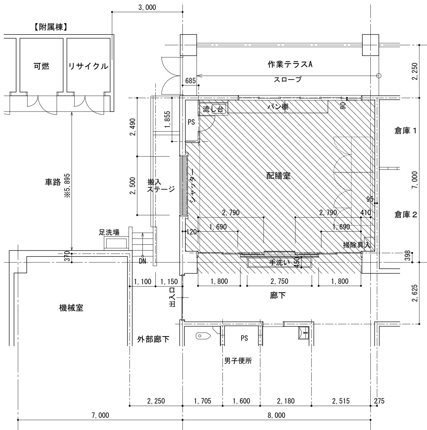
既存平面図
