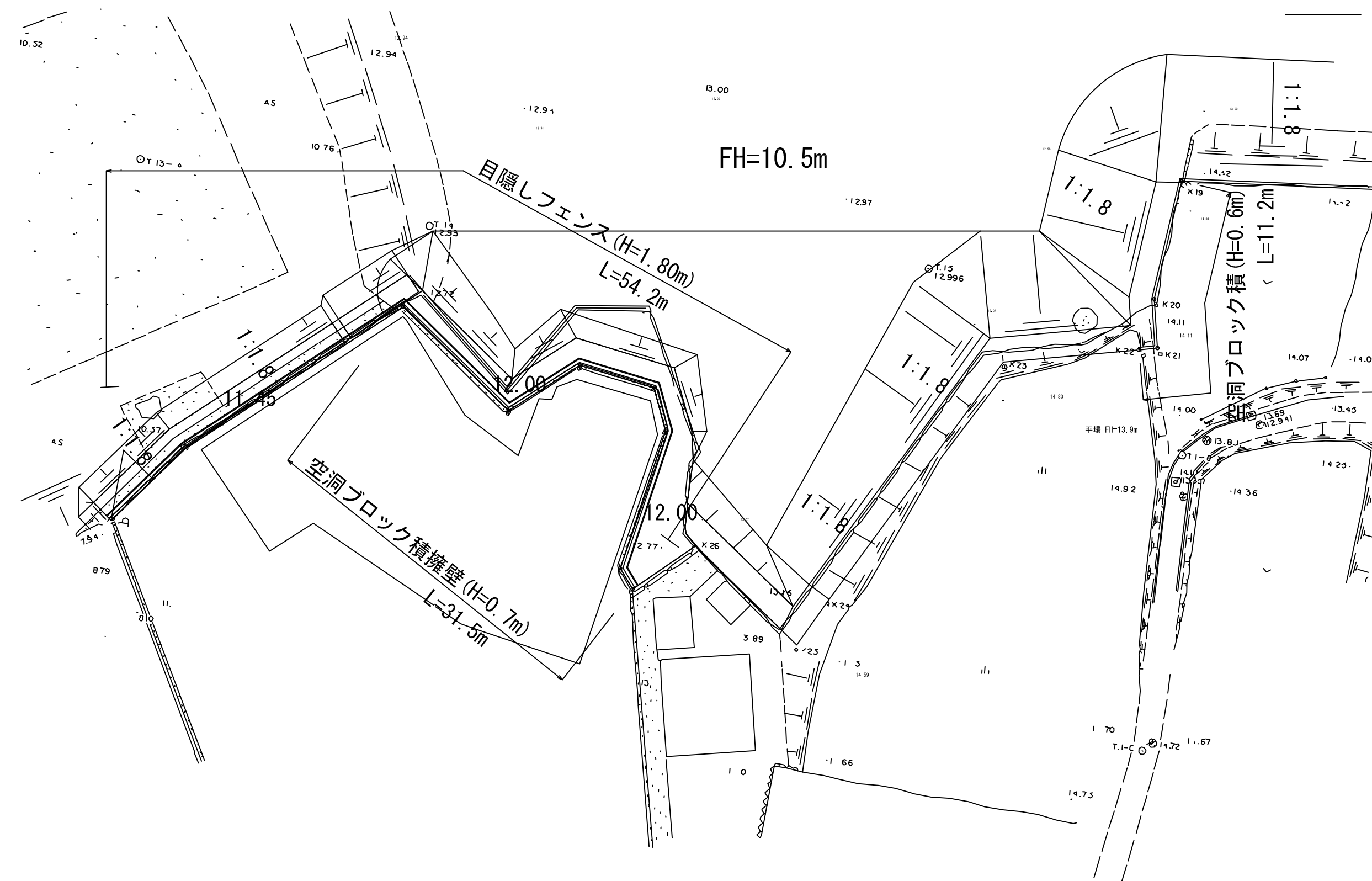
平面図 S=1:500
