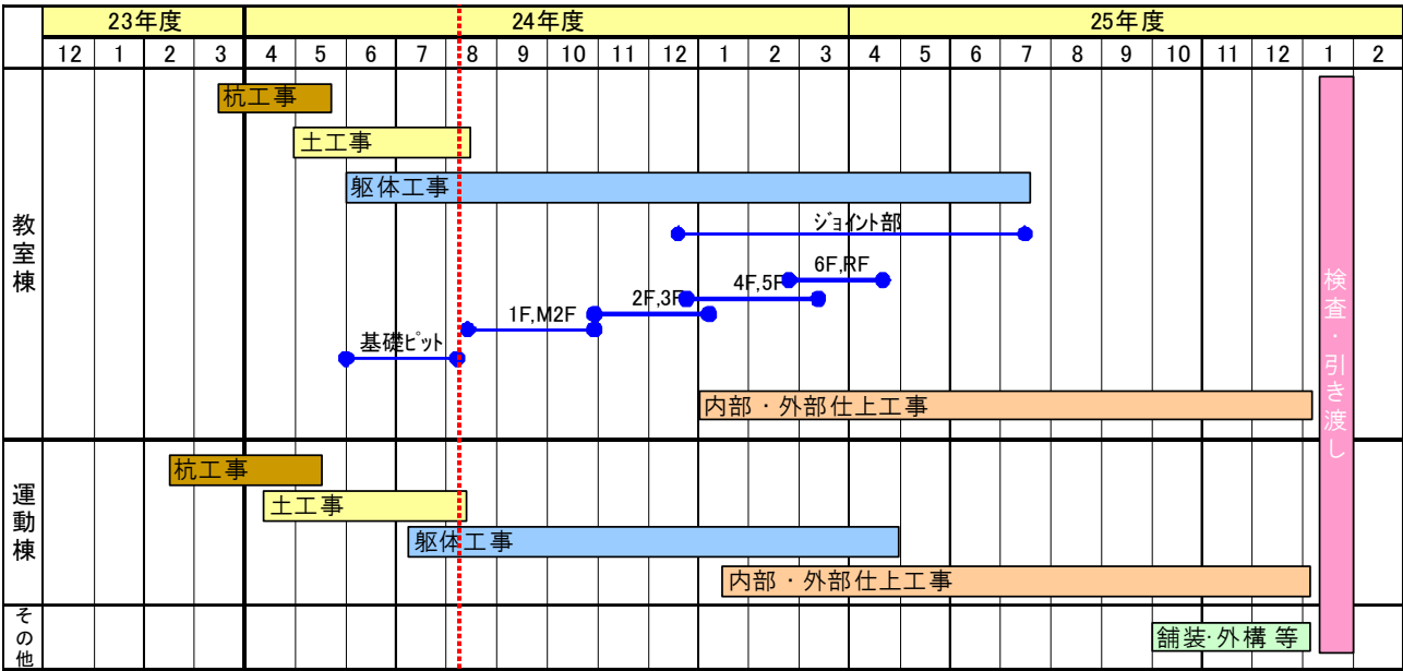
【現在の工事状況】敷地全景
