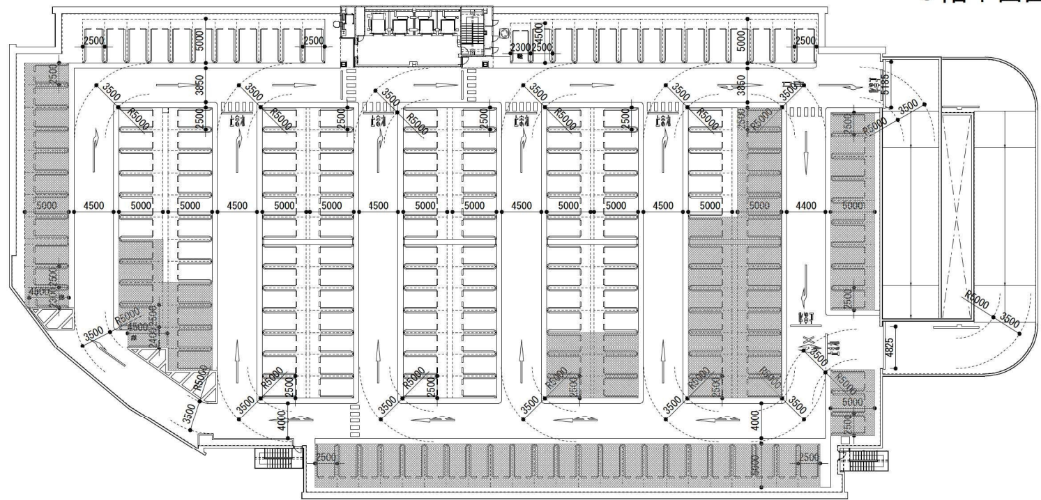
9階平面図
