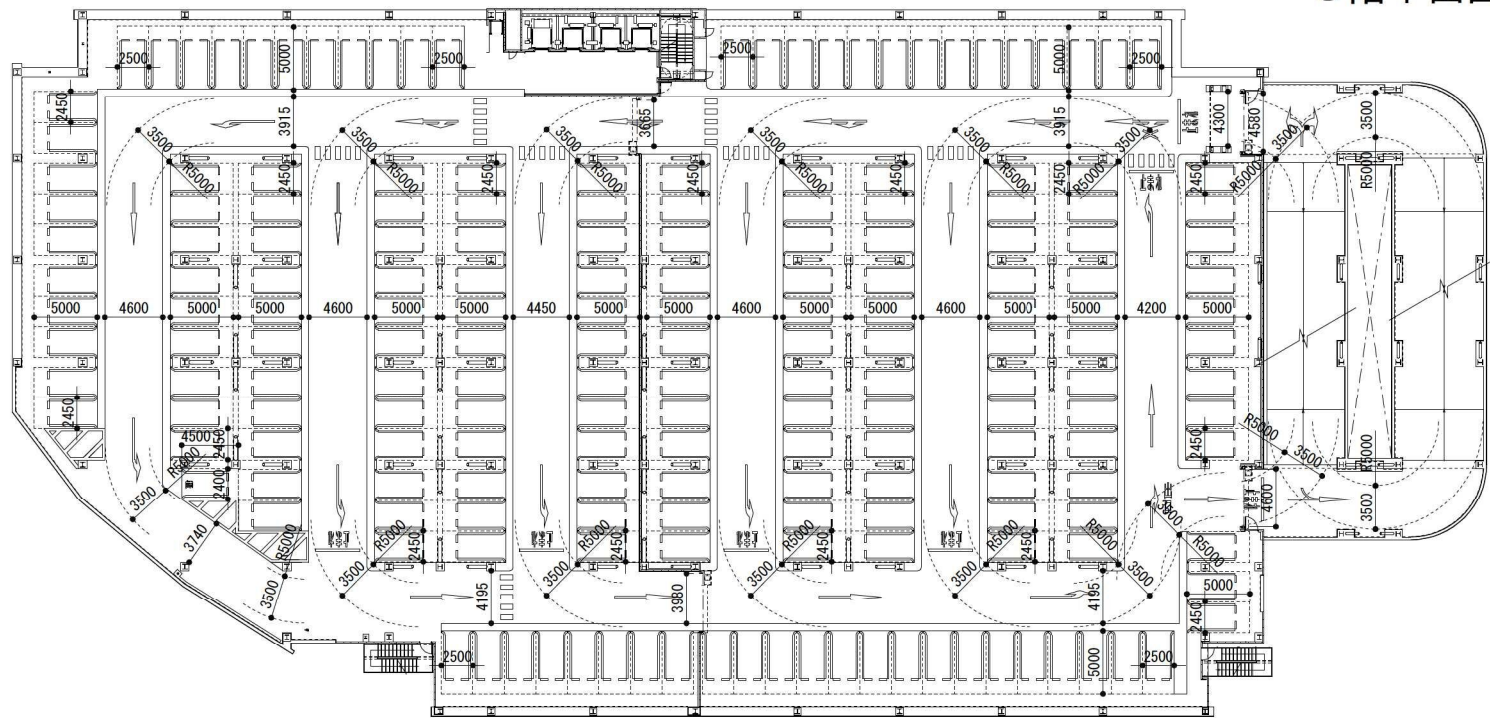
8階平面図
