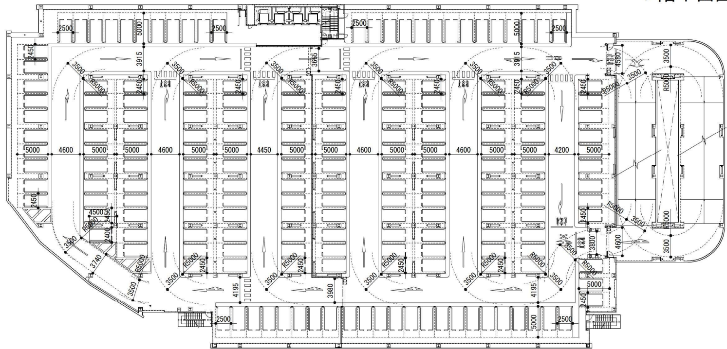
7階平面図
