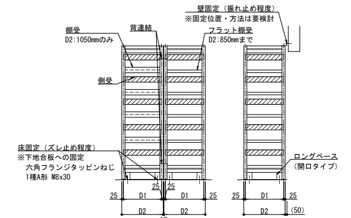
側面図 1/30
