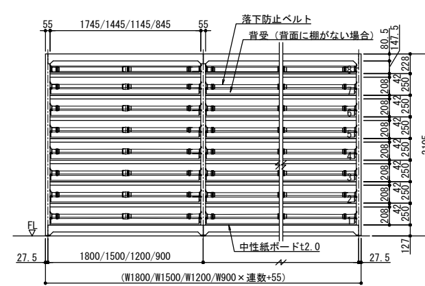
正面図 1/30
