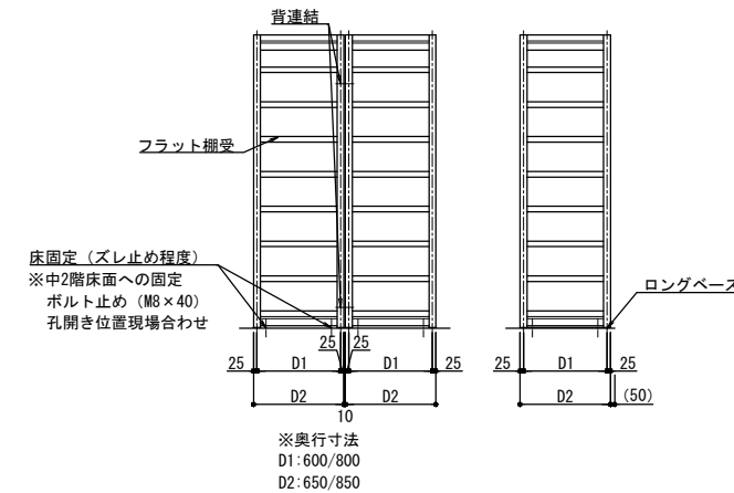
側面図 1/30
