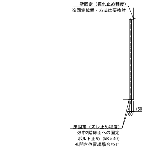
側面図 1/30
