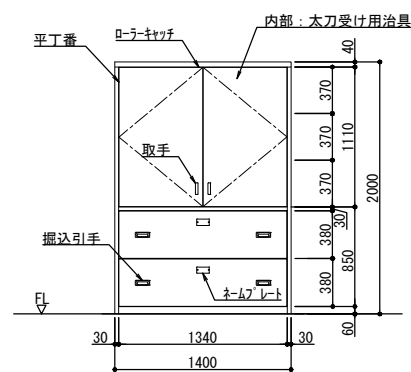
正面図 1/30
