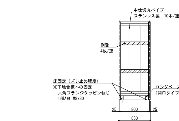
側面図 1/30
