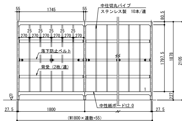
正面図 1/30
