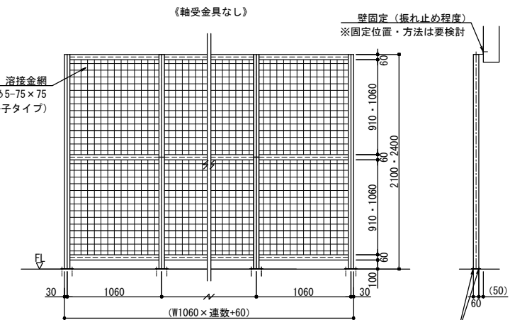
正面図 1/30
