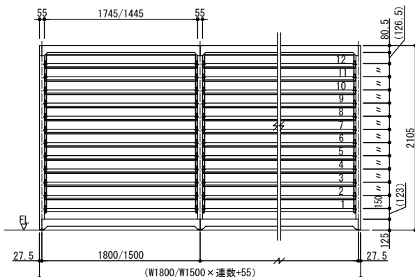
正面図 1/30
