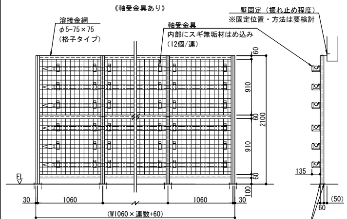
正面図 1/30
