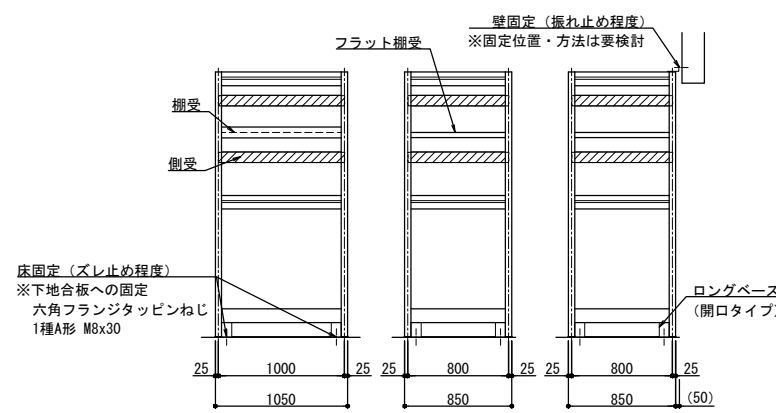
側面図 1/30
