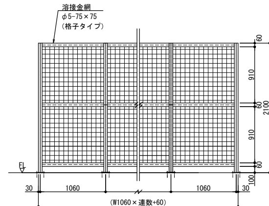
正面図 1/30
