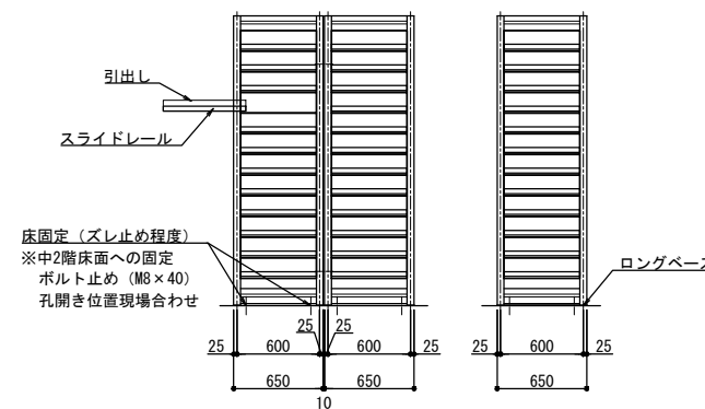
側面図 1/30
