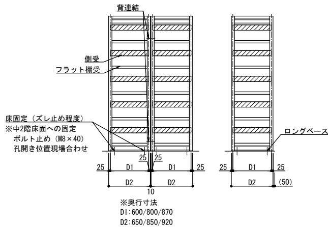
側面図 1/30
