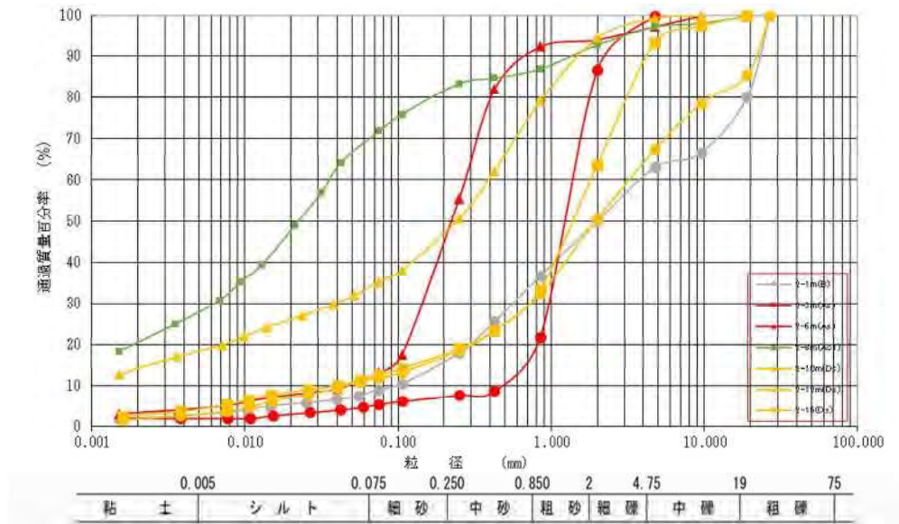
図 4.4.1 各層の粒径加積曲線
