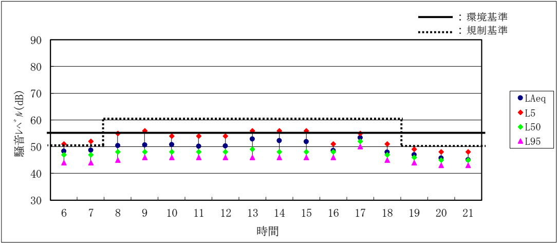
騒音レベルの時間変化
