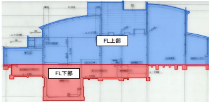
図 5.4.2 FL 上部・FL 下部の工事区分
