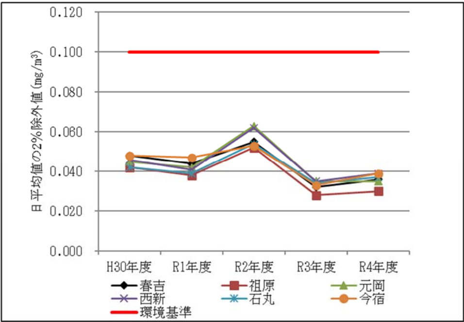
注：春吉局のデータの内、H30年度～R3年度は市役所局のデータを示す。 出典：「福岡市大気測定結果報告書」H30年度～R4年度版 福岡市環境局
