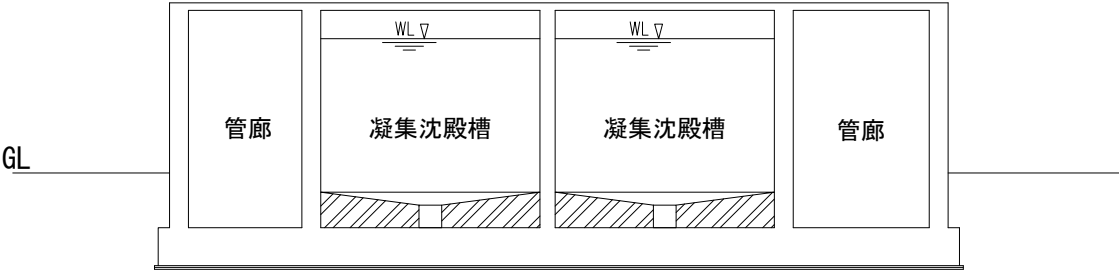
① - ① 断面図
