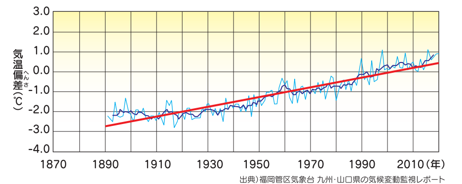
年平均気温の経年変化(福岡市)
