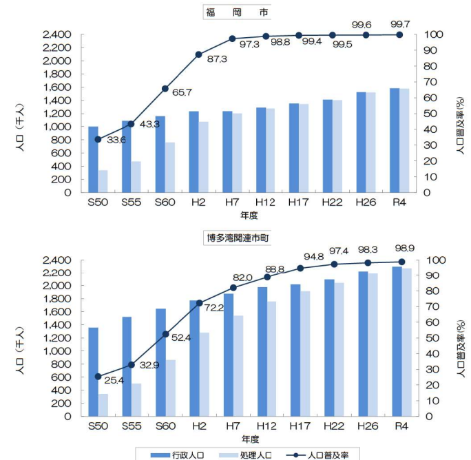
図 13 博多湾関連市町における下水道普及状況の推移
