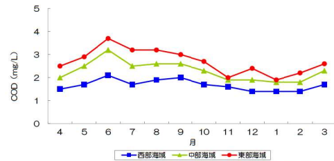
図 47 CODの季節変化（令和元年～令和5年度の全層※15カ年平均）
