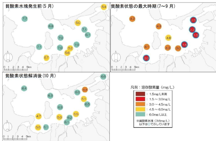
図 26 海底上 0.1m の溶存酸素量(DO)の分布(令和5年度)
