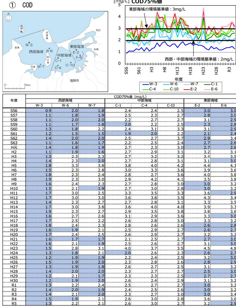
図27 COD全層平均値の75%値の推移と環境基準の達成状況
