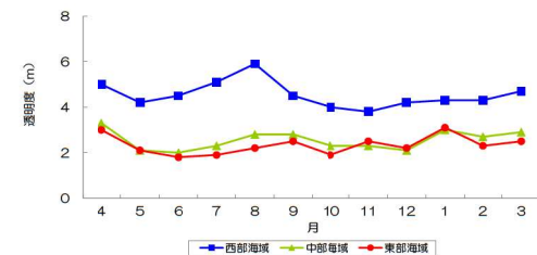
福岡市水質測定結果報告書（福岡市環境局）、令和5年度博多湾水底質調査委託報告書（福岡市環境局）をもとに作成 図 56 透明度の季節変化（令和元年～令和5年度の5ヵ年平均）
