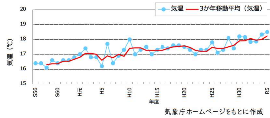
図 5 気温(福岡管区気象台)の推移
