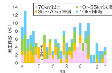
九州海域の赤潮（水産庁九州漁業調整事務所）をもとに作成 図 65 赤潮発生規模別の件数の推移
