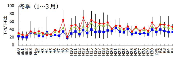
図 37 T-N/T-P 比（モル比）の経年変化
