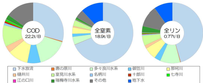
図16 博多湾への流入負荷の内訳(令和元年度)
