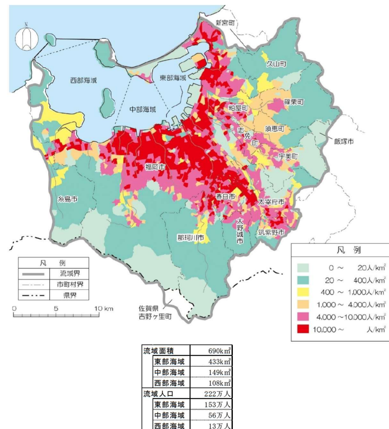
図11 博多湾流域の面積と人口密度分布
