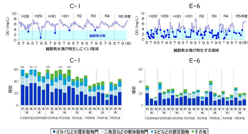
図 34 貧酸素水塊の発生前後における底生生物の種数の比較(平成 28~令和 5 年度)
