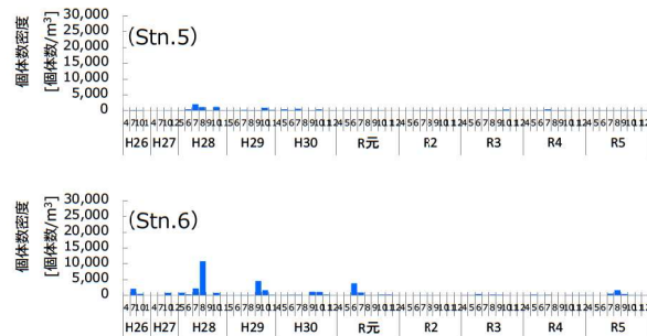
福岡市農林水産局の提供データをもとに作成 図 89 (2) アサリ浮遊幼生の個体数密度の経年変化
