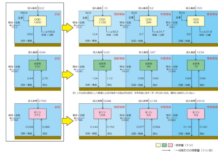
図 78 博多湾のCOD、全窒素、全リンの收支(令和元年度)
