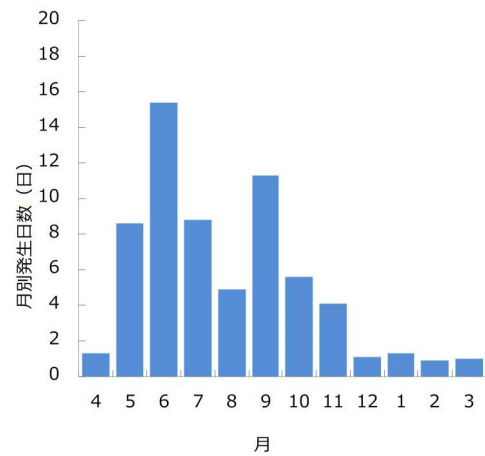
九州海域の赤潮（水産庁九州漁業調整事務所）をもとに作成 図 63 赤潮の月別発生日数（平成28年度～令和5年度の平均値）
