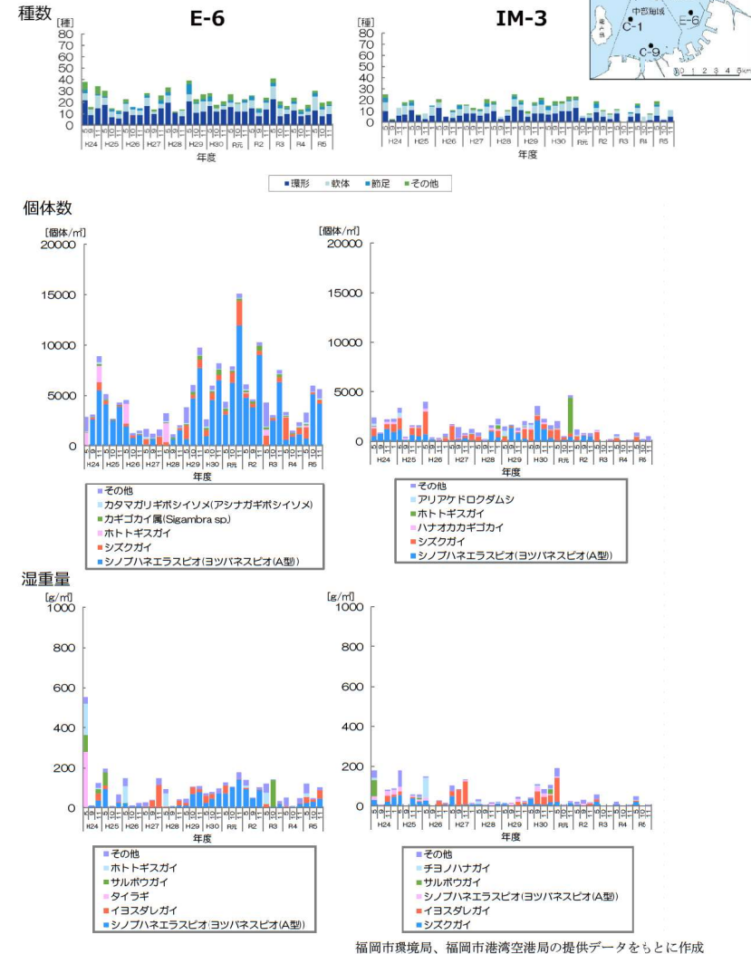
図 98 底生生物の種数・個体数・湿重量の経年変化
