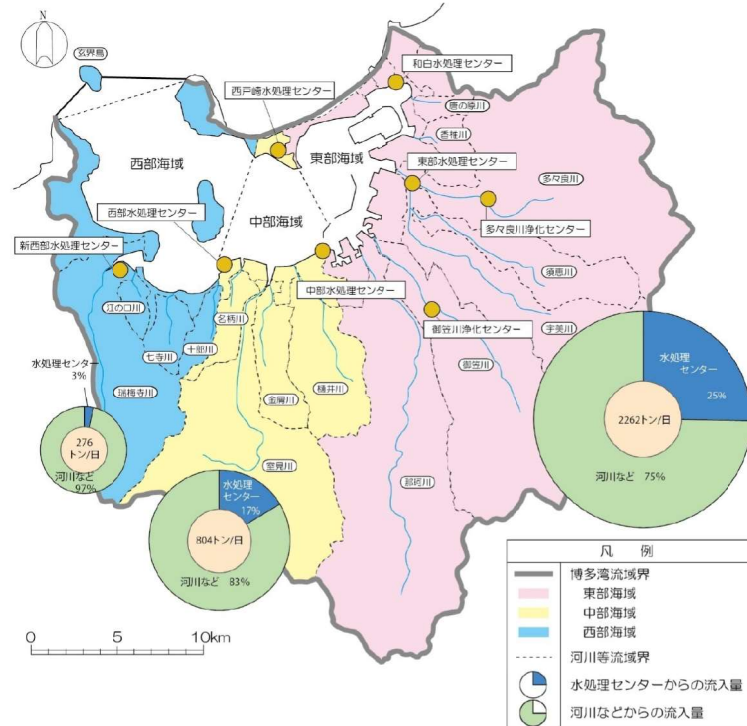
図 12 博多湾に流入する主な河川と水処理センター・浄化センターの位置及び流入量
