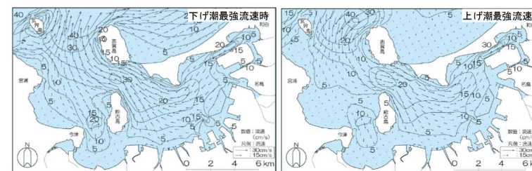
図10 博多湾の流向・流速
