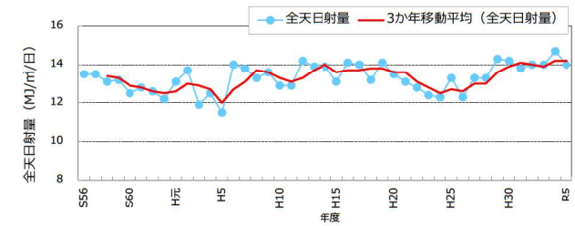
図 8 全日射量(福岡管区気象台)の推移
