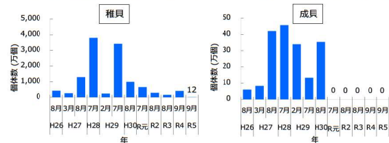
注) 図中の個体数は多々良川河口干潟全体の推定個体数です。 福岡市農林水産局の提供データをもとに作成 図 91 多々良川河口干潟におけるアサリ稚貝・成貝の個体数の推移
