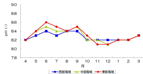
福岡市水質測定結果報告書（福岡市環境局）、 令和5年度博多湾水底質調査委託報告書（福岡市環境局）をもとに作成 図 60 pHの季節変化（令和元年～令和5年度の表層 ※25 カ年平均）
