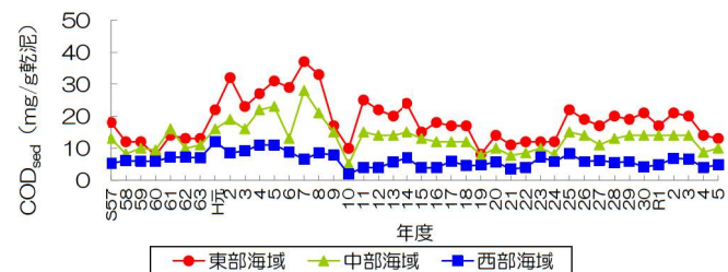
福岡市水質測定結果報告書（福岡市環境局）、 令和5年度博多湾水底質調査委託報告書（福岡市環境局）をもとに作成 図 69 底質のCOD sed の経年変化
