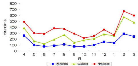
福岡市水質測定結果報告書（福岡市環境局）、令和5年度博多湾水底質調査委託報告書（福岡市環境局）をもとに作成 図 55 DIN/DIP 比（モル比）の季節変化（令和元年～令和5年度の表層5ヵ年平均）
