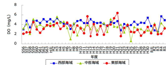
図 42 DO（底層※1年最低値※2）の経年変化
