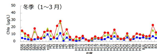
図 40 クロロフィル a (Chl a) (3層※平均) の経年変化
