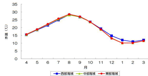
福岡市水質測定結果報告書（福岡市環境局）、 令和5年度博多湾水底質調査委託報告書（福岡市環境局）をもとに作成 図 59 水温の季節変化（令和元年～令和5年度の表層 ※15 カ年平均）
