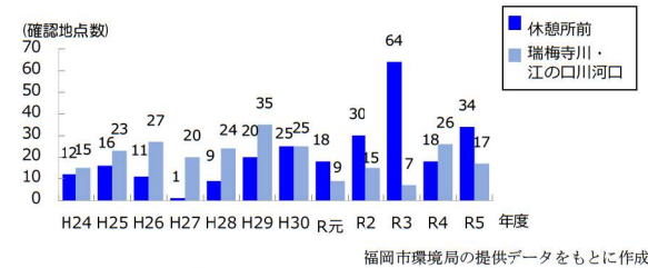
図 84 カブトガニの卵塊の確認地点数の経年変化
