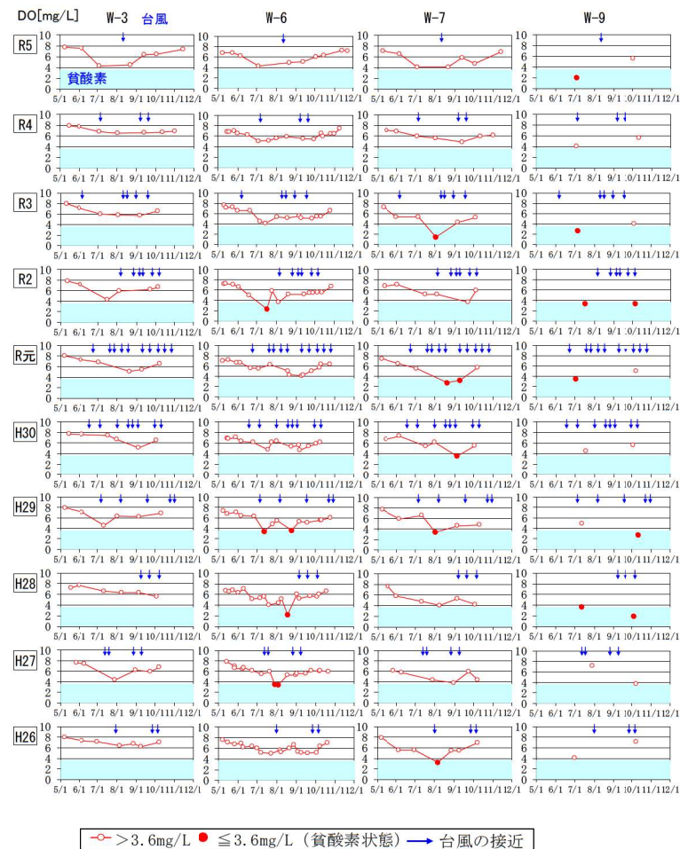
図 77(1) 底泥直上の溶存酸素量の経年変化
