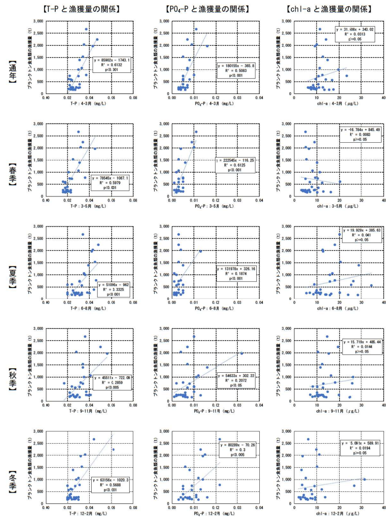
図 111 リン及び chl-a とプランクトン食魚類の漁獲量の関係
