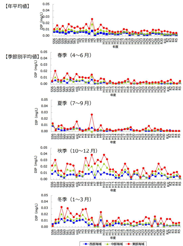
福岡市水質測定結果報告書（福岡市環境局）、 令和5年度博多湾水底質調査委託報告書（福岡市環境局）をもとに作成 図 36 溶解性無機態リン（DIP）（表層※平均）の経年変化
