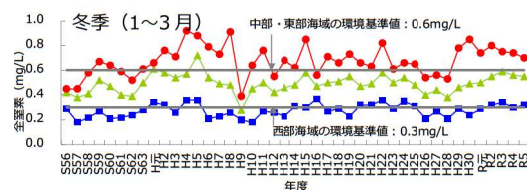
図33 全窒素（表層※平均）の経年変化
