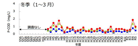
図32 懸濁性COD (P-COD) ※ 1 (3層 ※ 2 平均) の経年変化
