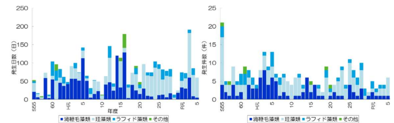
九州海域の赤潮（水産庁九州漁業調整事務所）をもとに作成 図 64 赤潮発生延べ日数（左）、赤潮発生延べ件数（右）の推移
