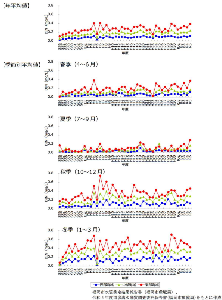
図 35 溶解性無機態窒素（DIN）（表層※平均）の経年変化
