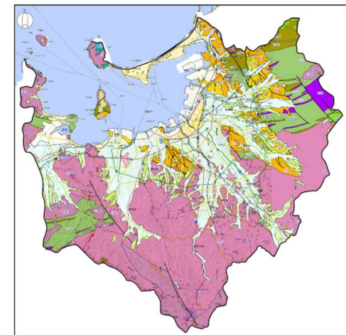
図 13 博多湾流域の地質図
