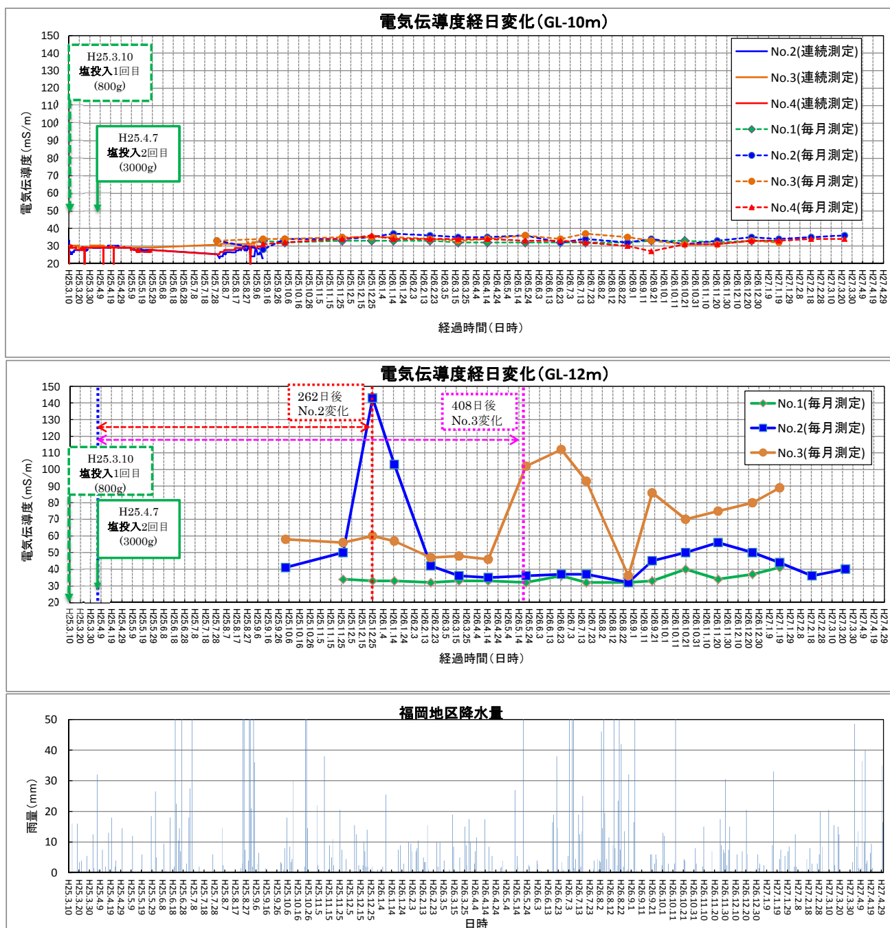
図8 春住小学校 流向・流速試験（トレーサー試験）結果
