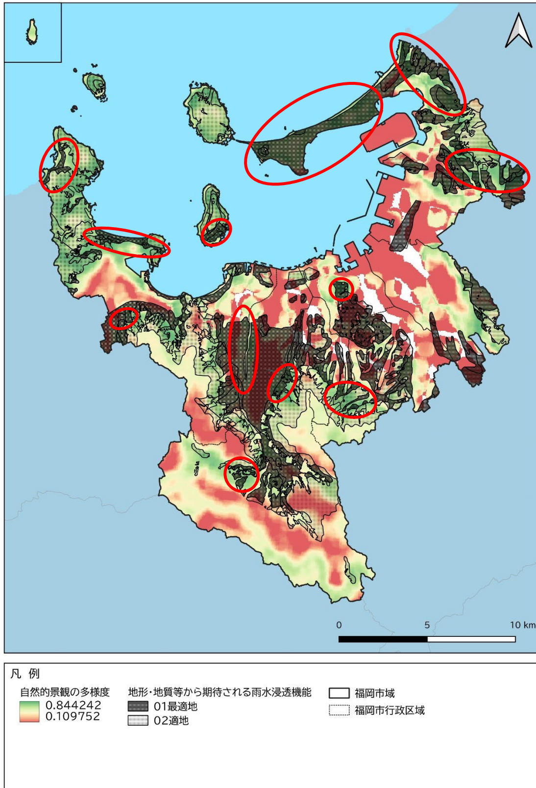
図 95 自然的景観の多様度×地形・地質等から期待される雨水浸透機能 【雨水の浸透が期待でき、生物多様性保全上も重要な場所を評価する場合】
