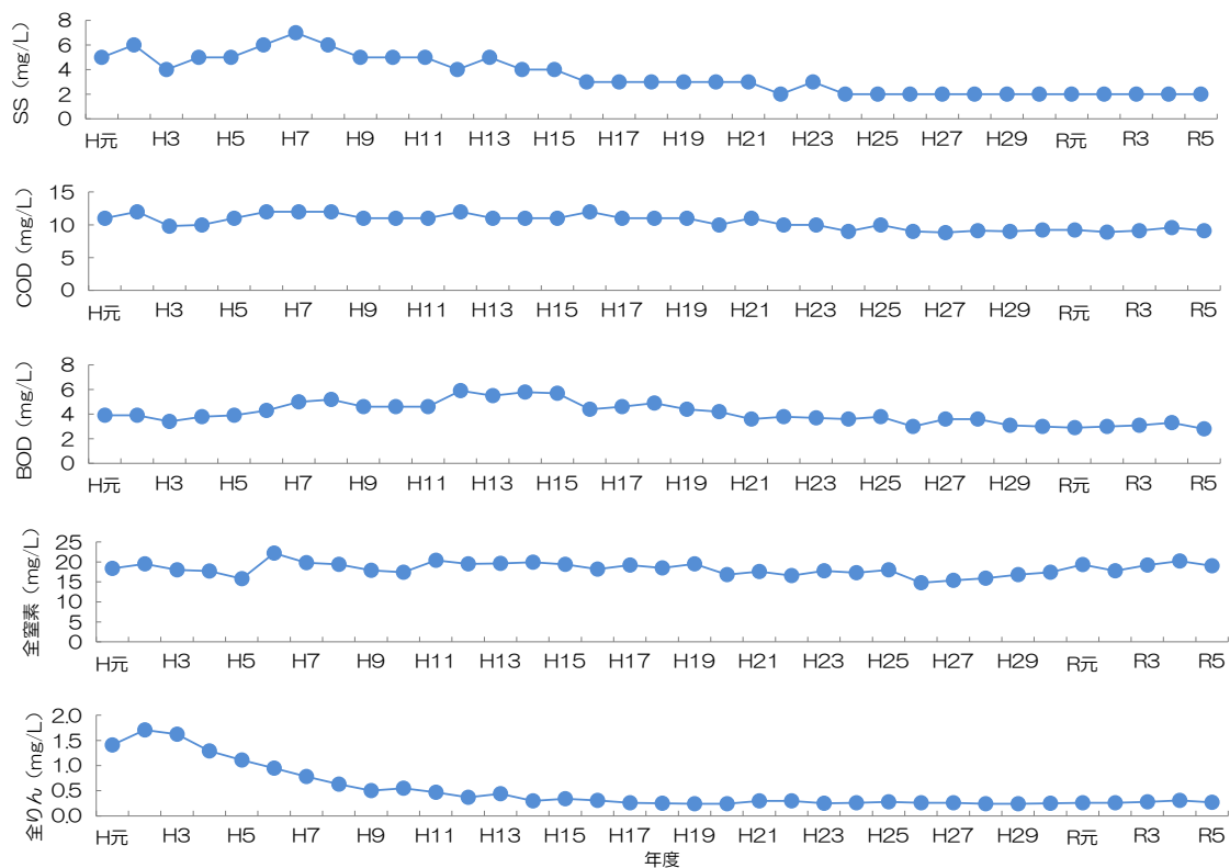
図 22 福岡市における水処理センター放流水質の推移（全センターの平均値）
