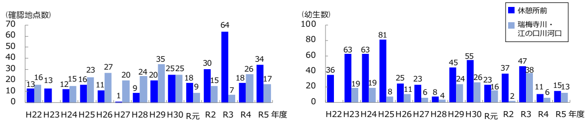
図 32 今津干潟におけるカブトガニの卵塊確認地点数(左)と幼生数(右)の経年変化
