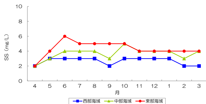
図 62 懸濁物質（SS）の季節変化（令和元年～令和5年度の表層 ※5 カ年平均）
