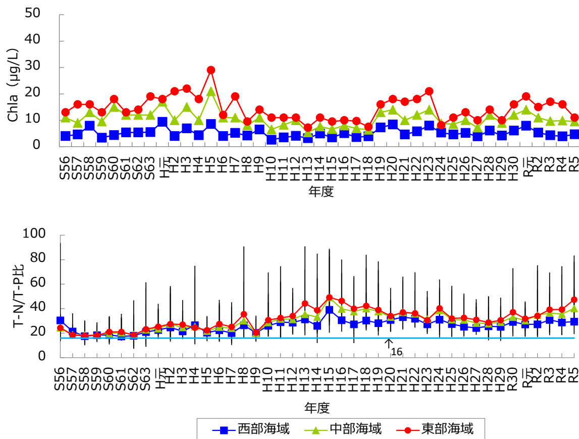
図 24 クロロフィル α(3 層平均) (上)と T-N/T-P 比(モル比) (下)の経年変化
