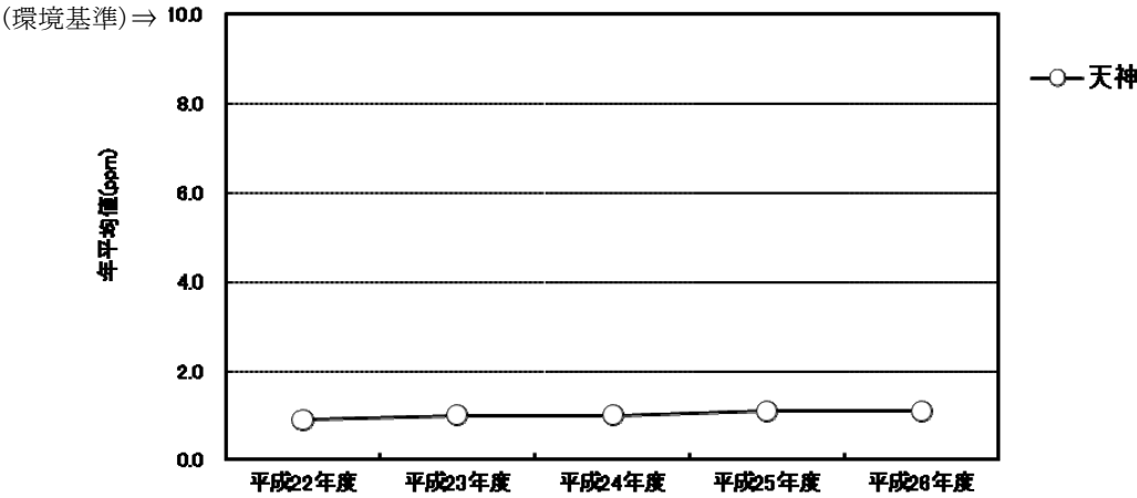
図 4.1.1-6 一酸化炭素の年平均値の経年変化
