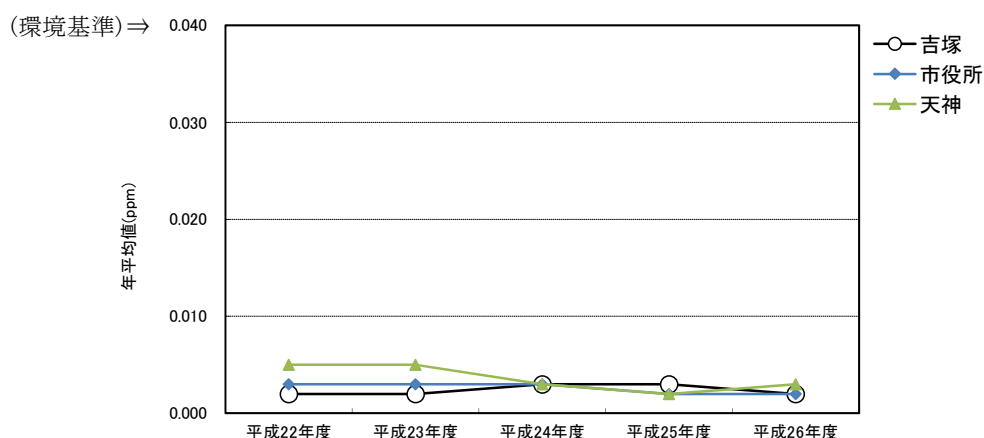
図 4.1.1-4 二酸化硫黄の年平均値の経年変化
