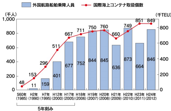
■博多港の外国航路乗降人員と 国際海上コンテナ取扱個数の推移
