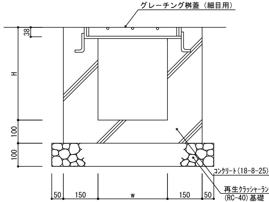
断面図
