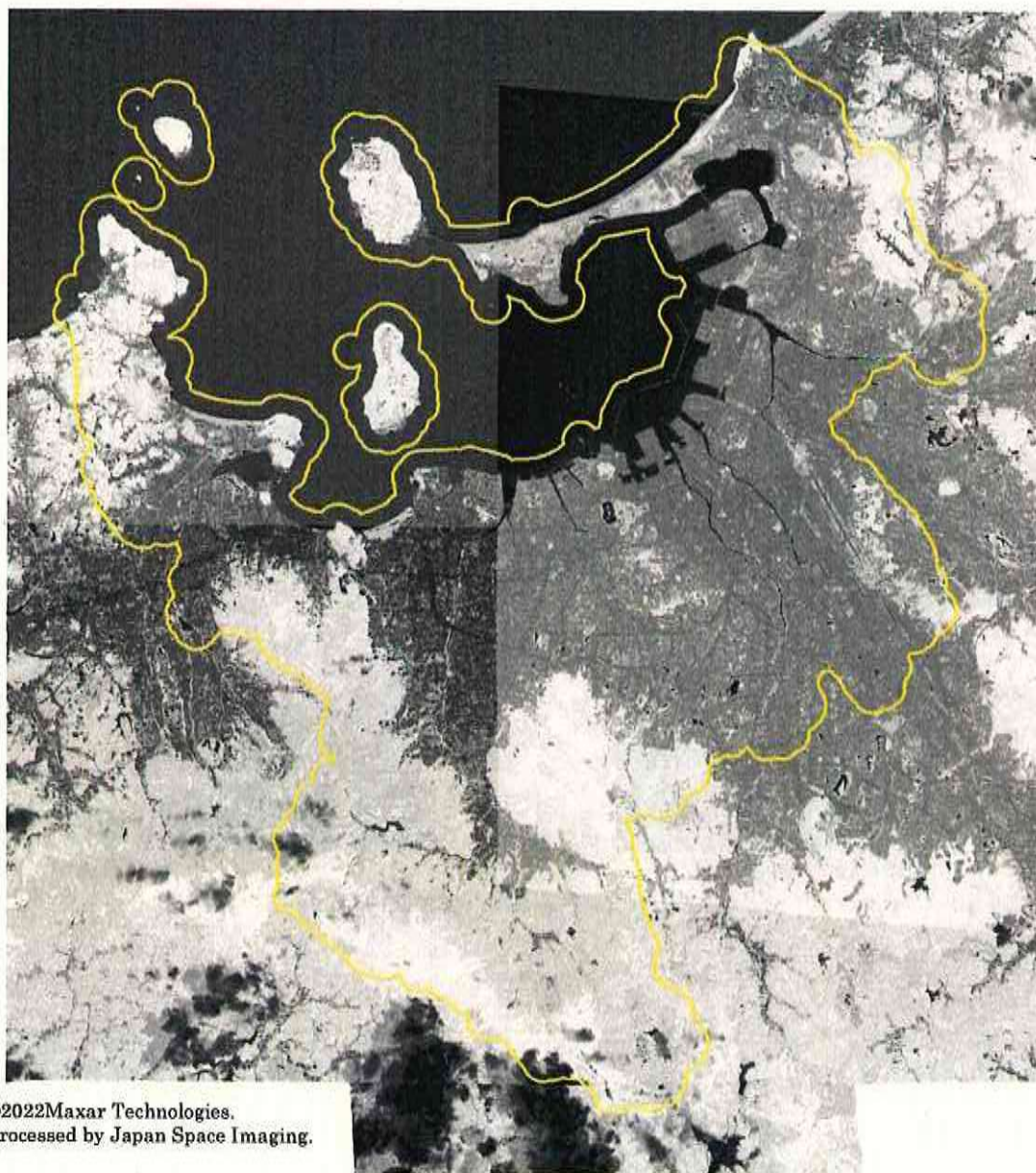
図 2-4 NDVI 画像
