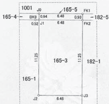
拡大図 縮尺:1/250
