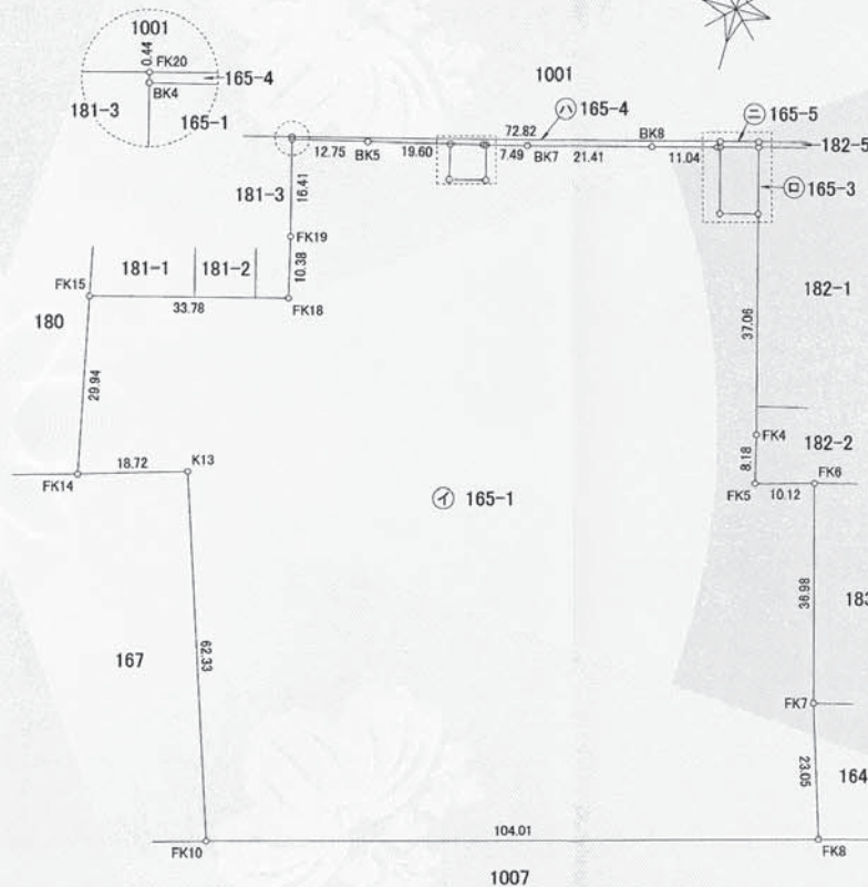
拡大図 縮尺:1/250
