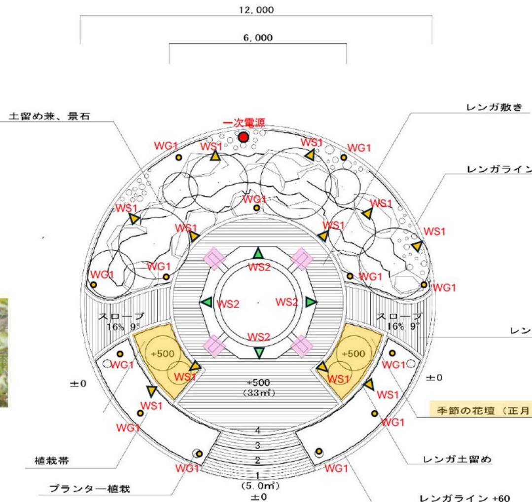
レンガ敷き
