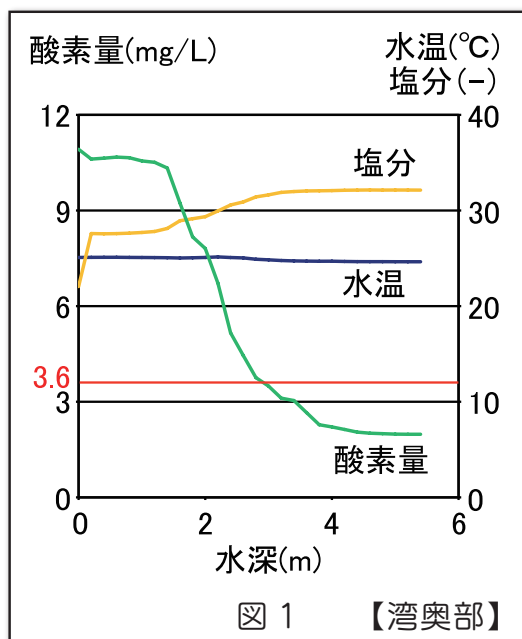
図 1：貧酸素水塊発生時の海面から海底までの水中の酸素量、塩分及び水温の変化（保健環境研究所による調査）
