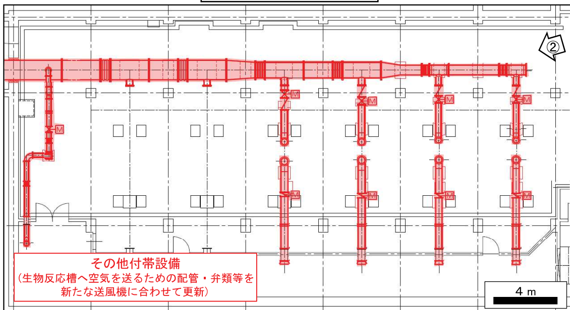
送風機棟地下 1 階 平面図
