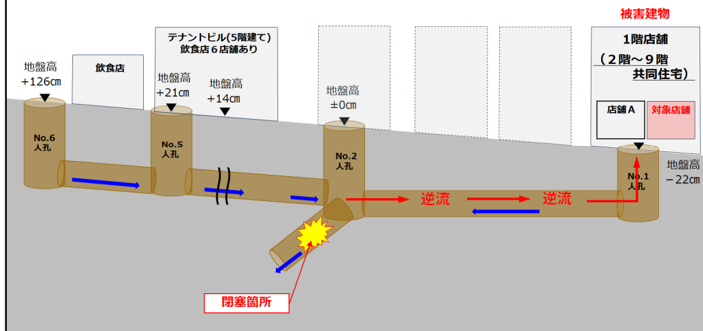
本管閉塞イメージ図（断面図） A-A
