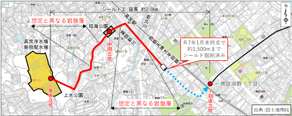
工事平面図
