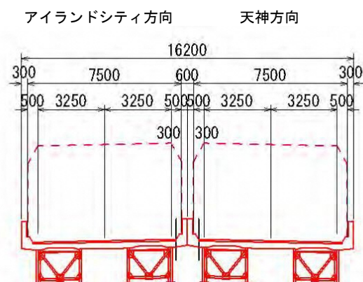
図 1-3-4 標準断面図
