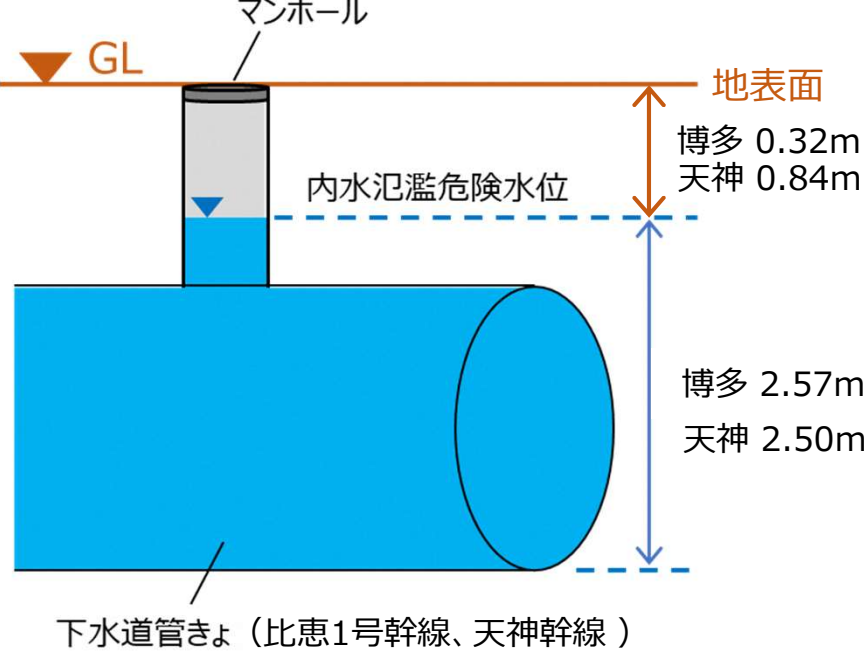
水位観測所における内水氾濫危険水位
