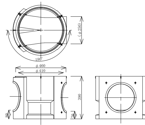
NRMC30 (C) -390 (250) 180 F (172.5° ~187.5°)
