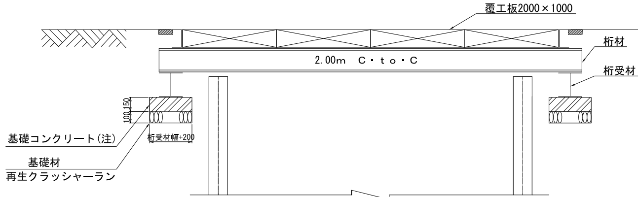
⑤覆工幅2.0~6.0m T-25荷重
