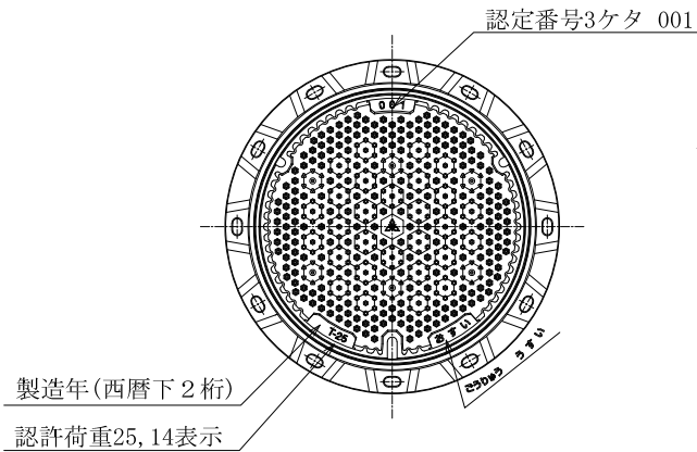
蓋表面図
