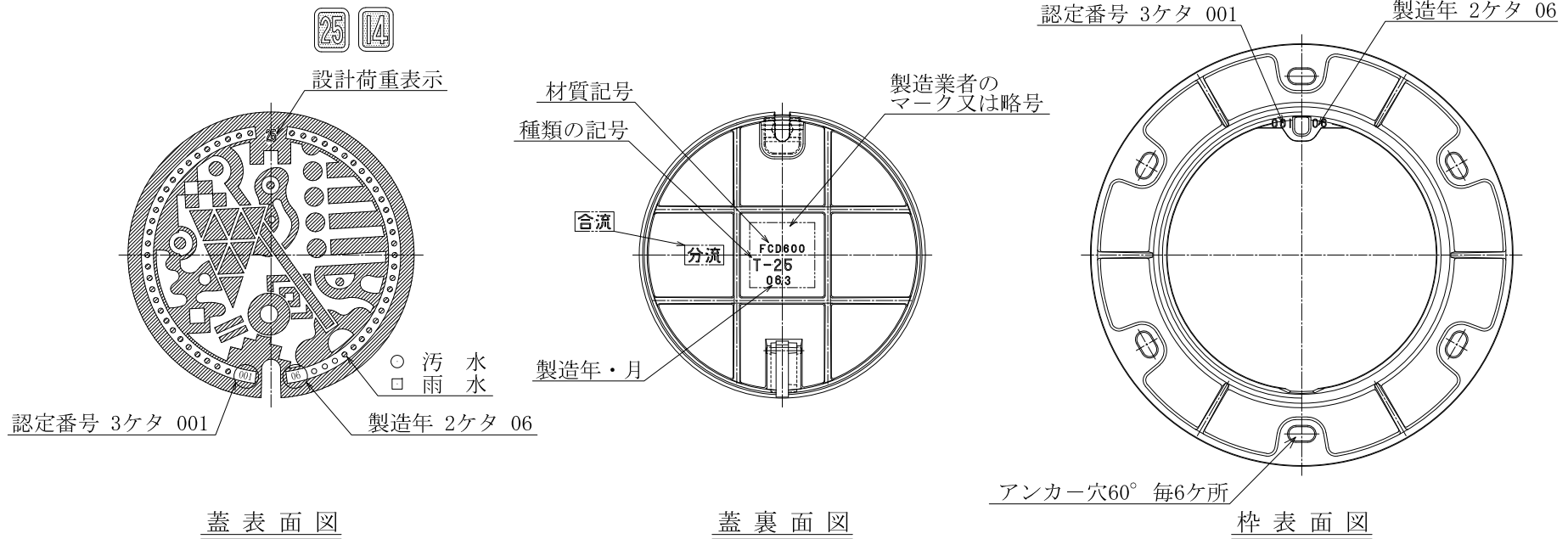
平面図
