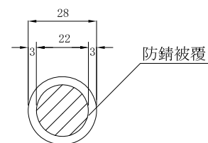
A-A 断面
