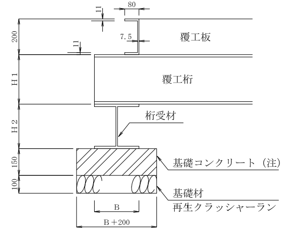
詳細図
