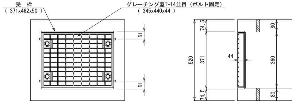
形状図 S = 1 : 15
