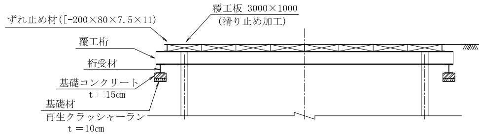
A-A 断面図
