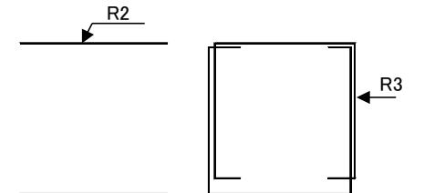
300mm以下鉄筋組立図
