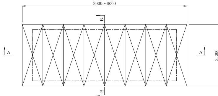
平面図
