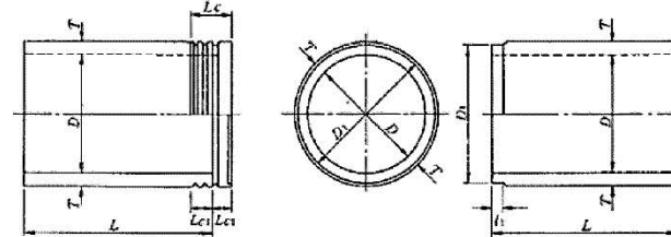
継手部詳細図
