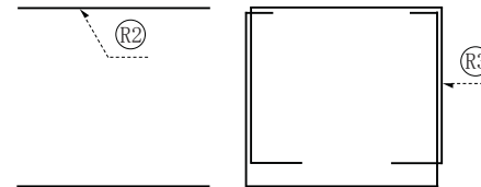
300mm 以下鉄筋組立図
