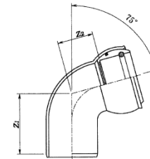
75度自在曲管 (略号 75SRF)
