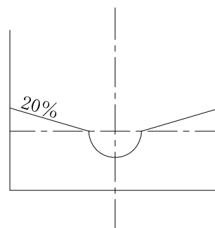
円形管のインバート
