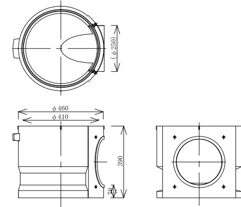
NRMC30 (C) -390 (250) キテン
