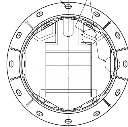
転落防止安全梯子付枠表面図
