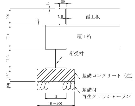
詳細図
