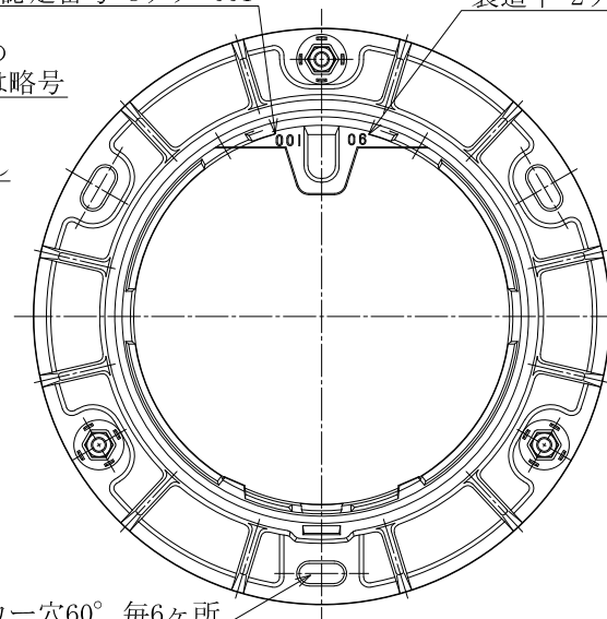
枠表面図
