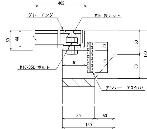
A部詳細図 S = 1 : 5
