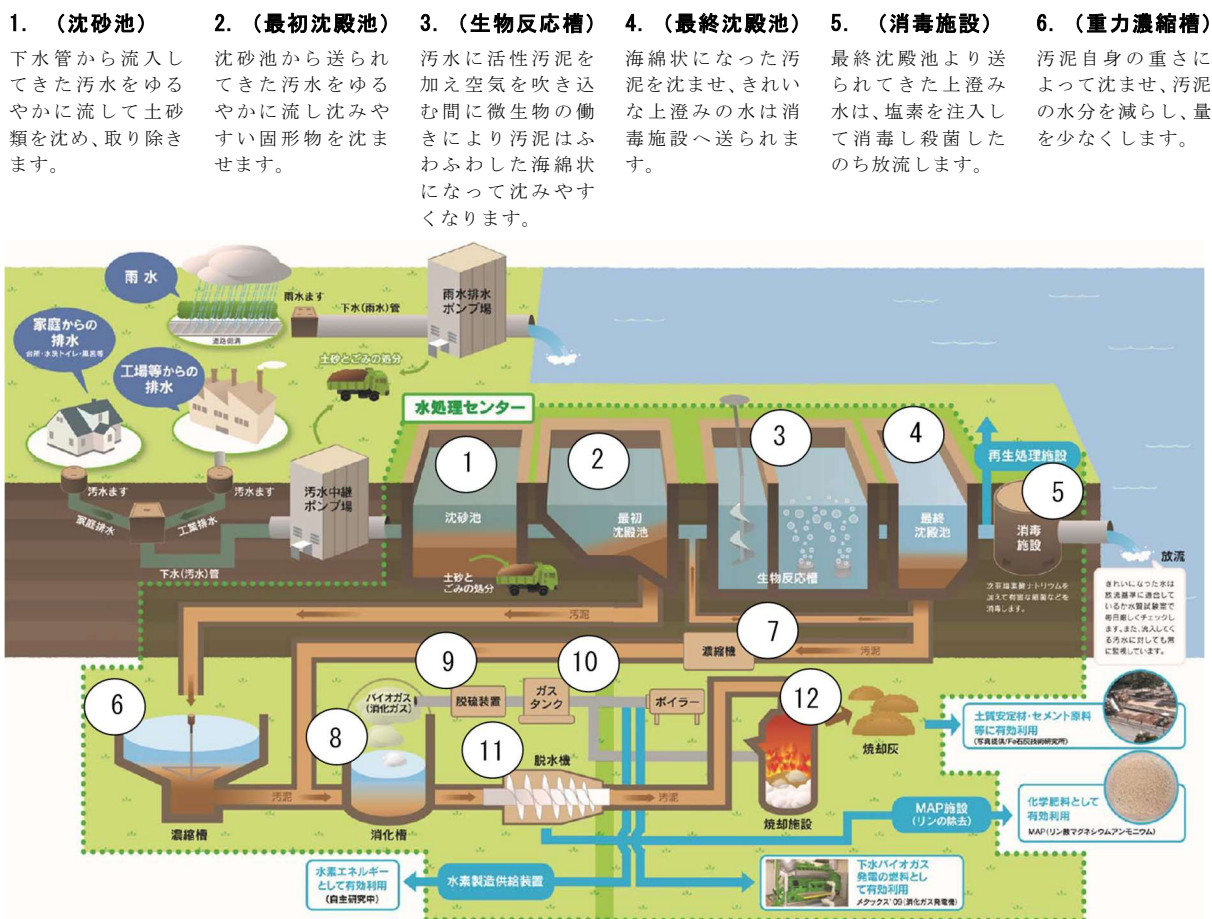
図 I - 2 処理場のしくみ
