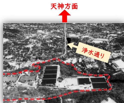
旧平尾浄水場(現福岡市植物園)
