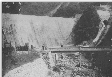
創設当時の曲洲ダム
