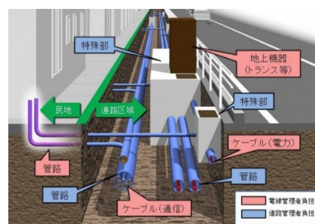
図一2 電線共同溝のイメージ
