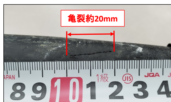
給水管(φ20mm)
