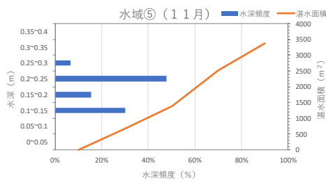
図 19 水域②～⑤ 月別水深頻度分布 (2019年4月～2022年8月) 注)池造成当初の水深が低い期間のデータ(2019年4月1～10日)は集計から除く
