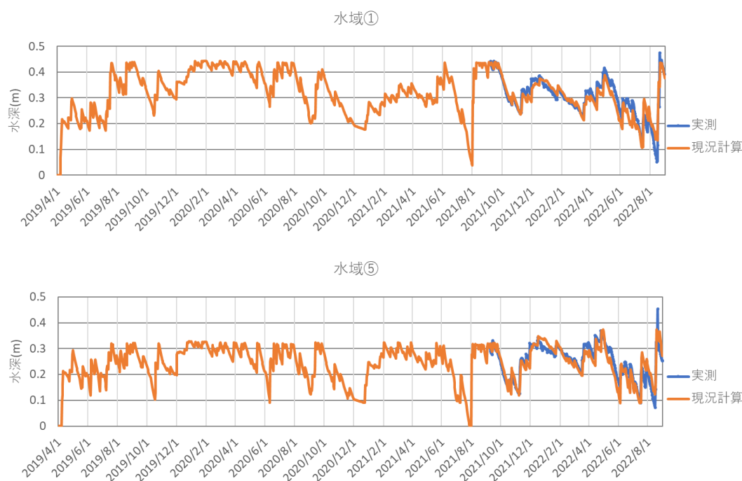
図 16 水深の現況計算結果
