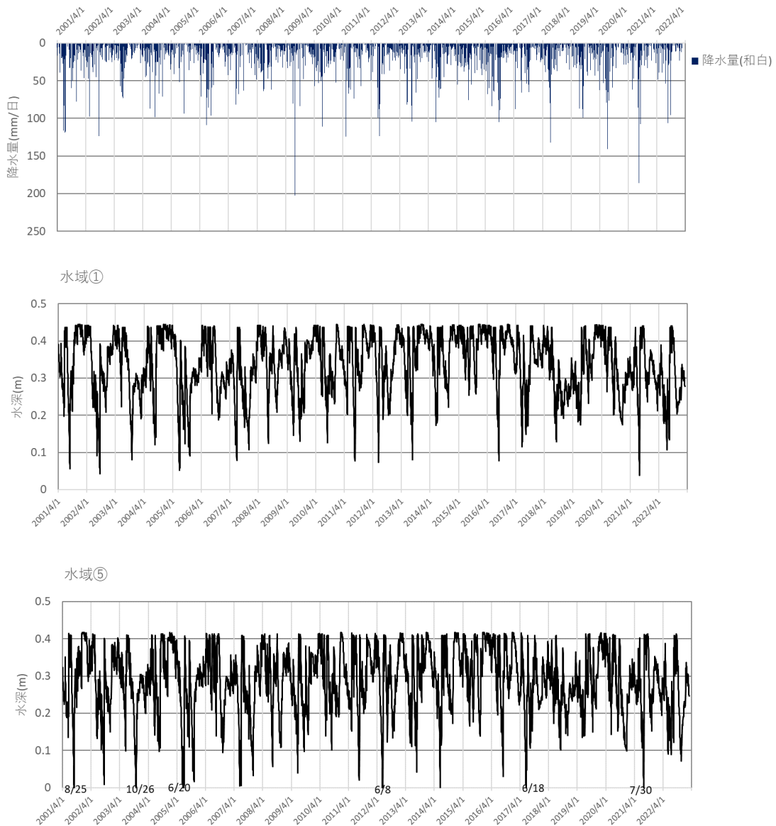
図 20 水位計算結果 (2001年4月～2023年2月)
