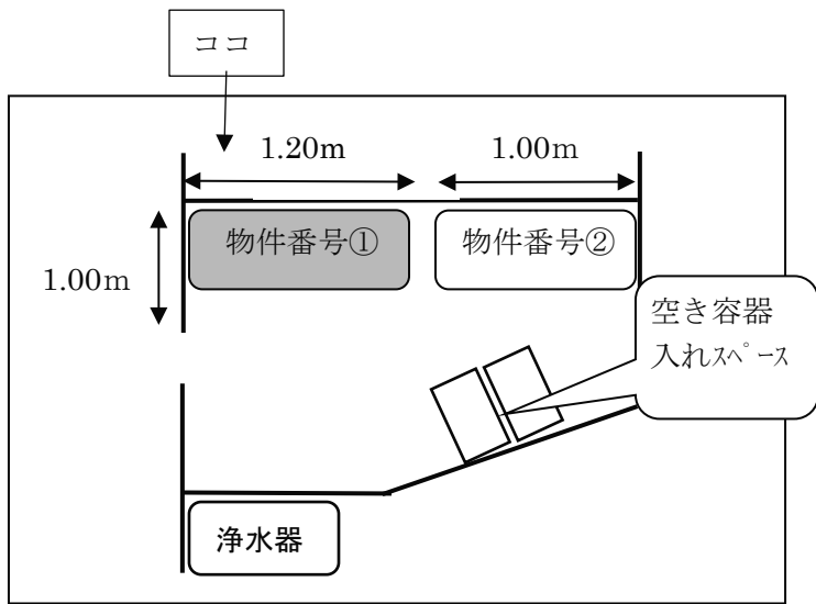
1階詳細図
