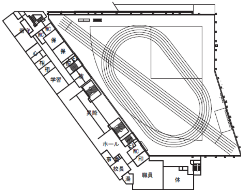
3階平面図
